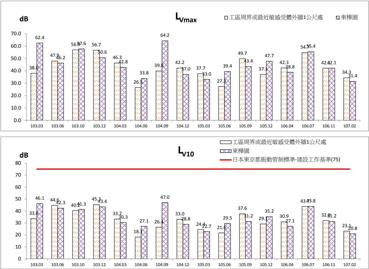
圖 2.2.4-1 營建振動監測結果圖
