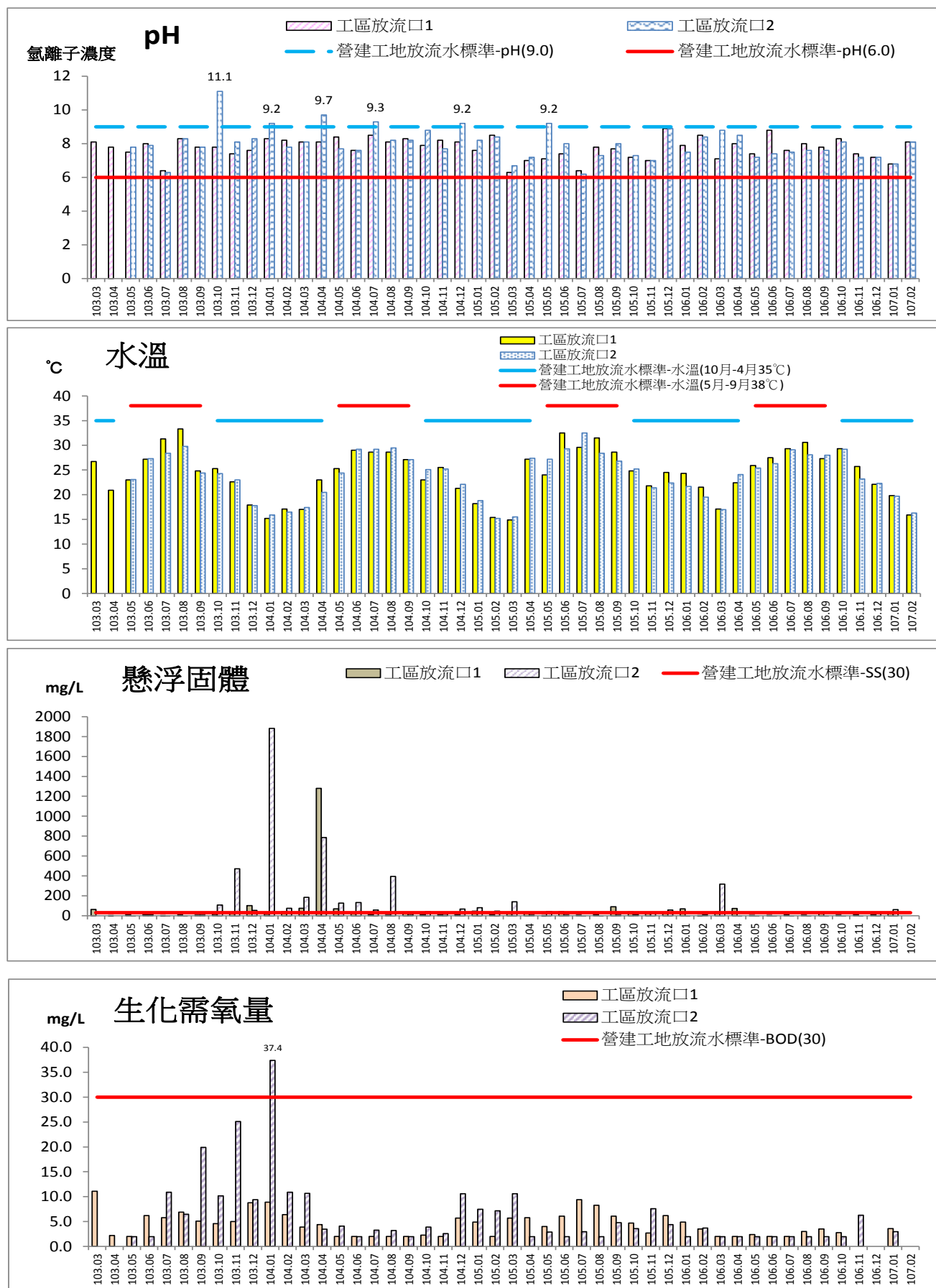
圖 2.6-1 放流水監測結果圖
