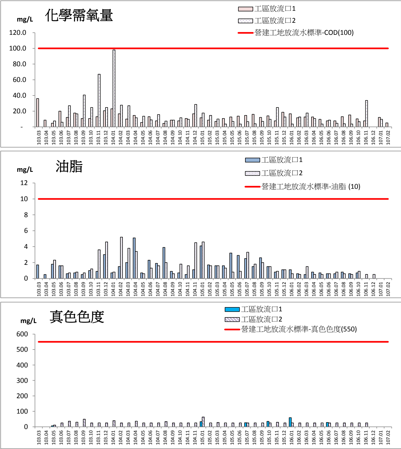
圖 2.6-1 放流水監測結果圖
