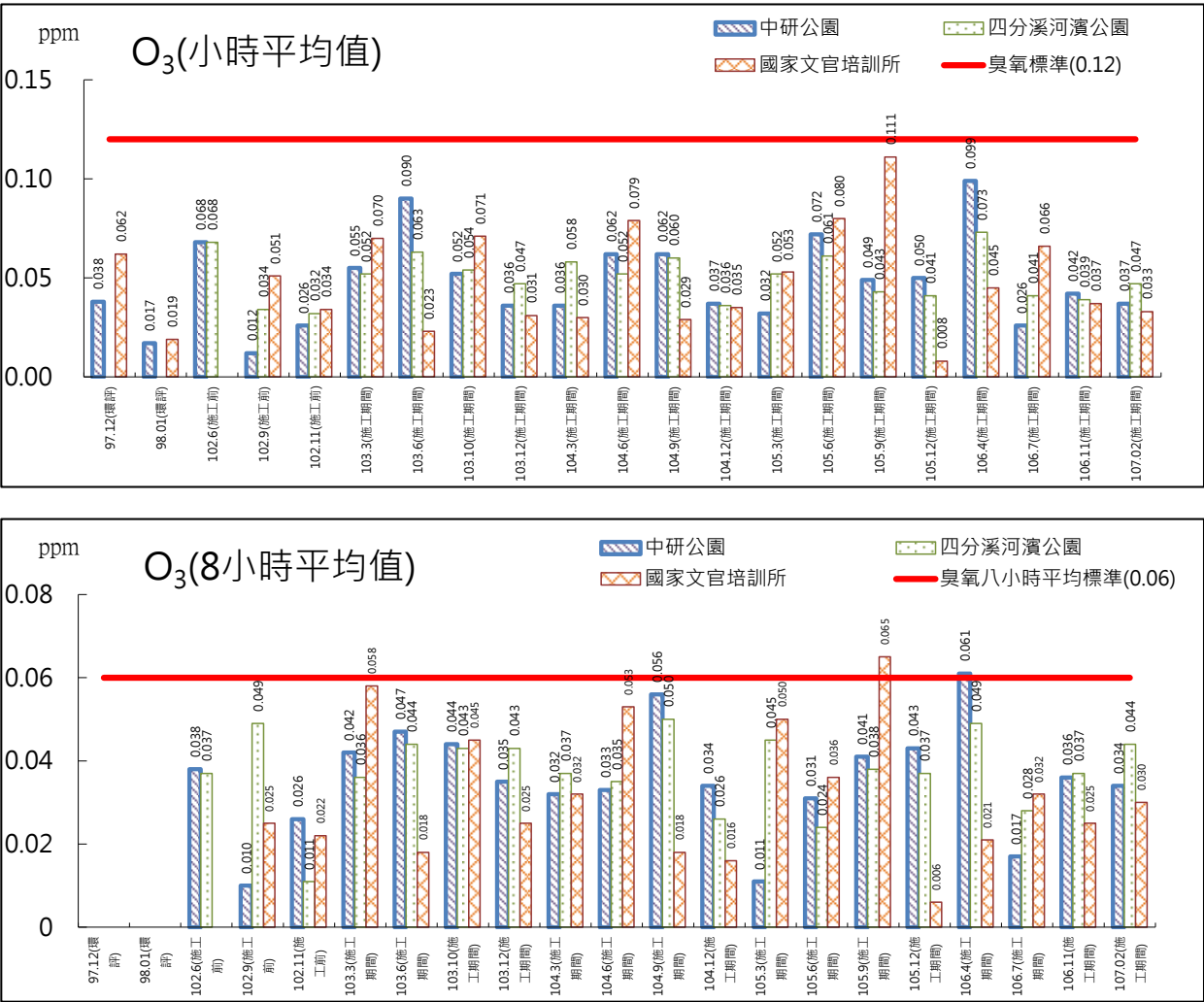
圖 2.1-1 空氣品質監測結果圖(續)
