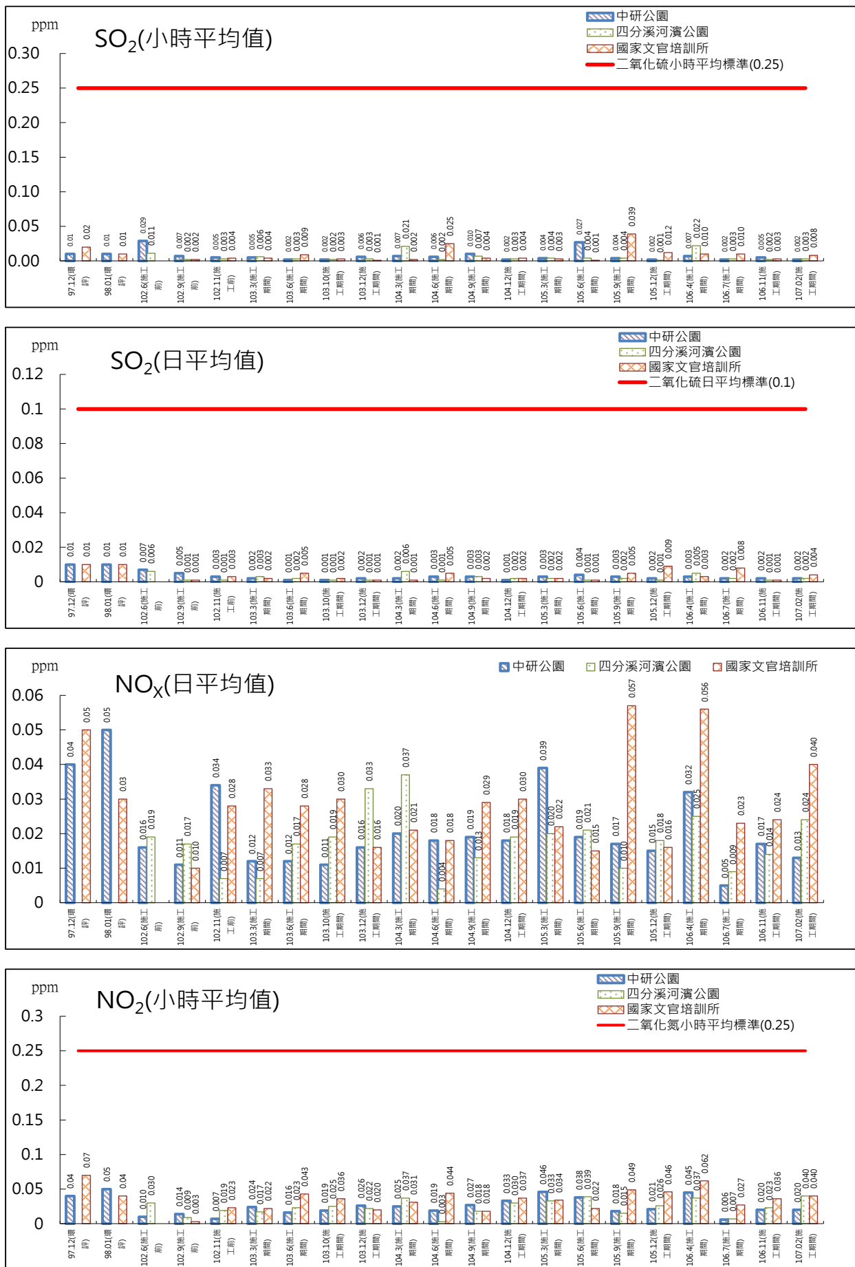
圖 2.1-1 空氣品質監測結果圖(續)
