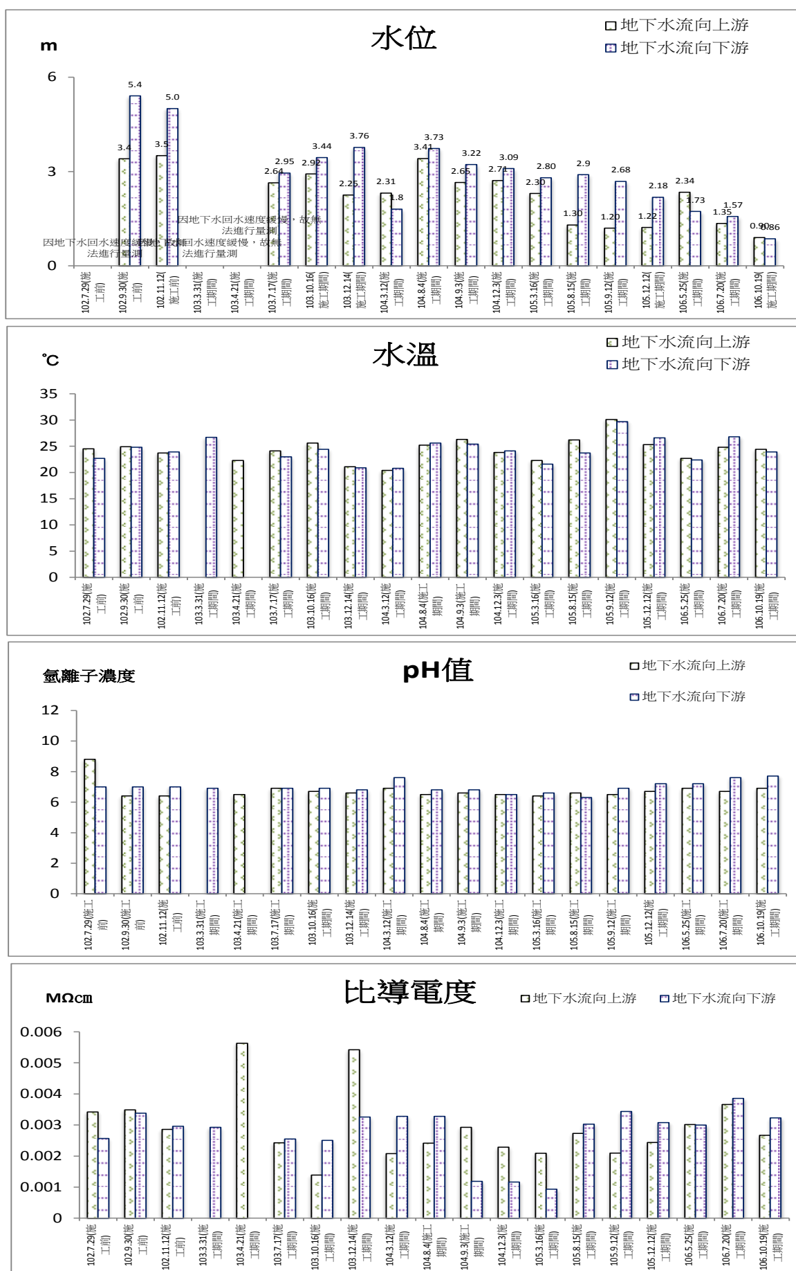
圖 2.5-2 地下水監測結果圖
