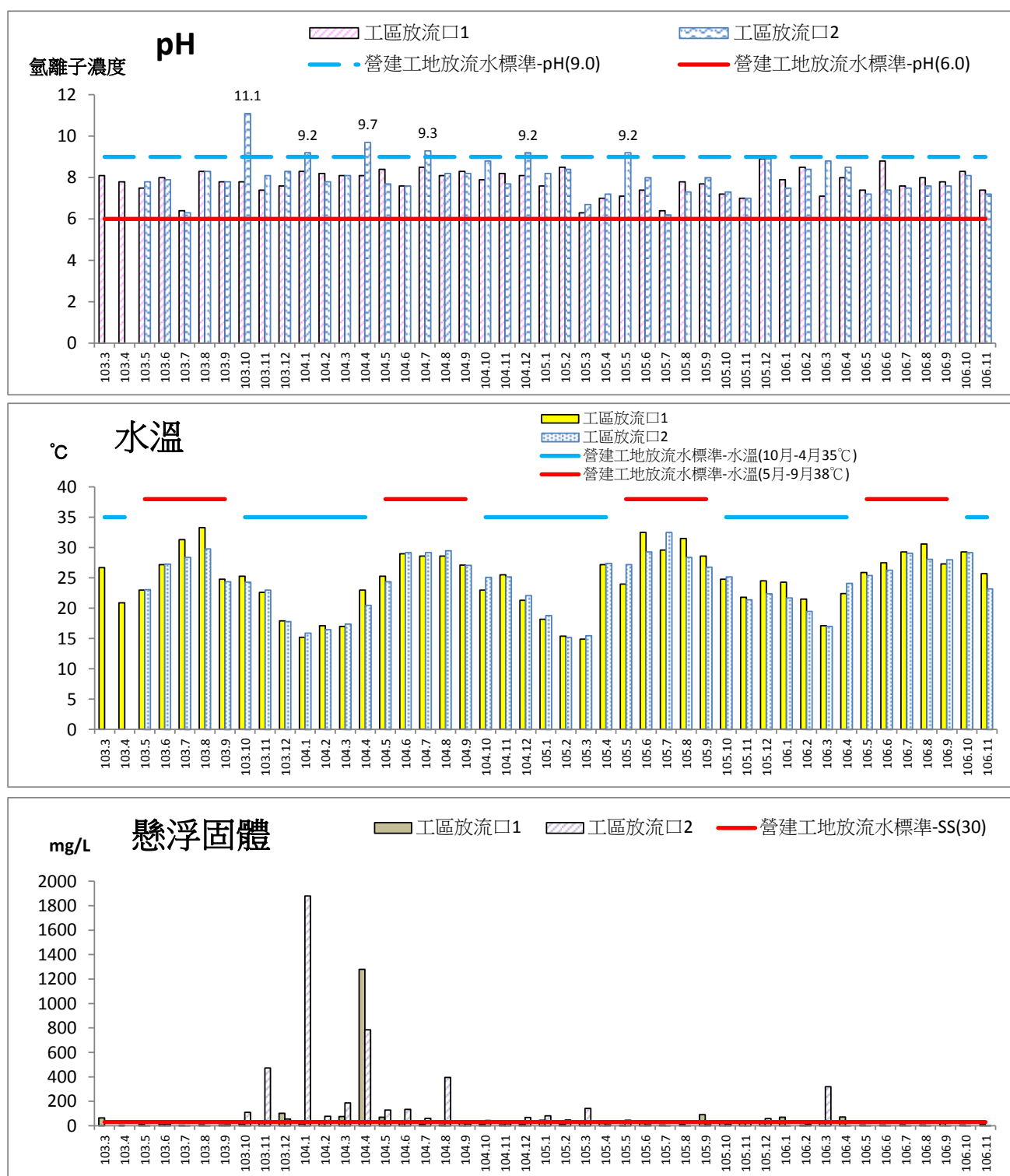
圖 2.6-1 放流水監測結果圖
