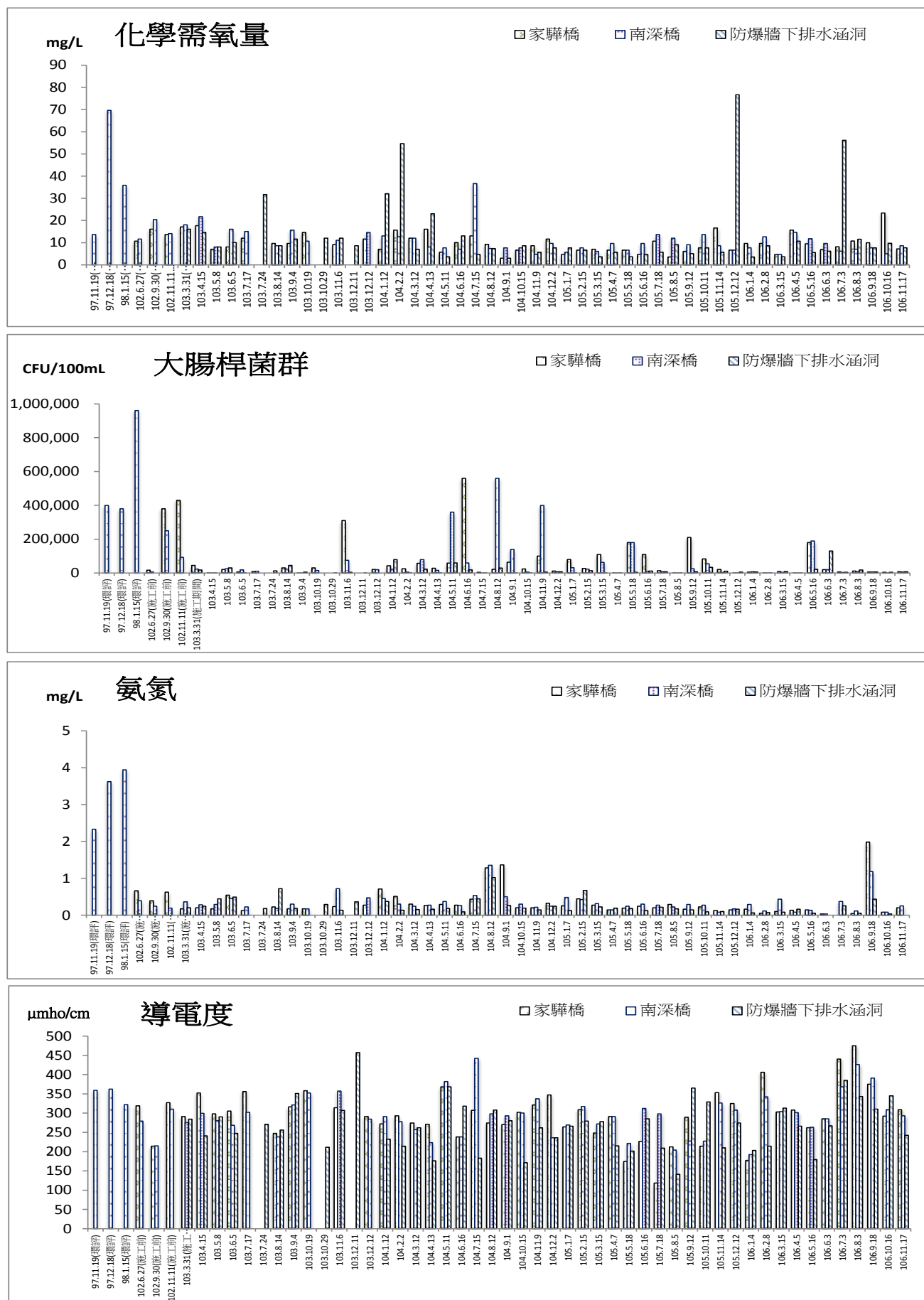
圖 2.4-2 地面水質監測結果圖(續)
