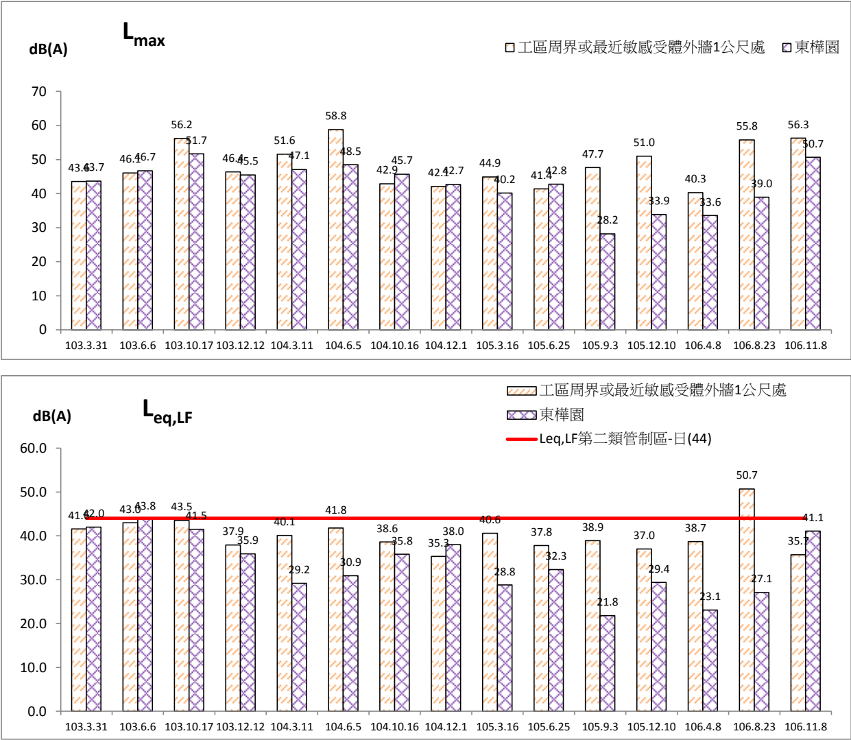
圖 2.2.5-1 低頻噪音監測結果圖
