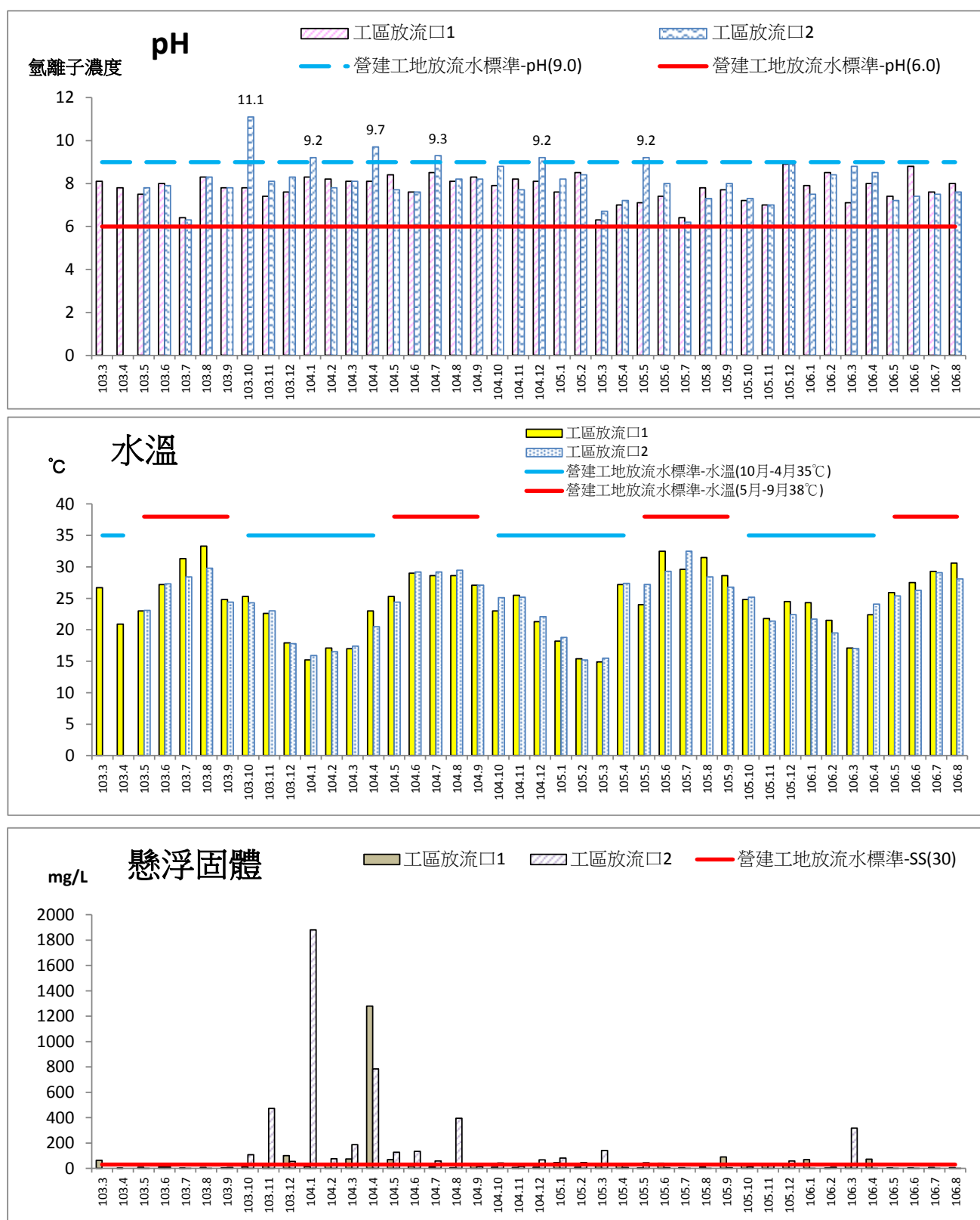
圖 2.6-1 放流水監測結果圖
