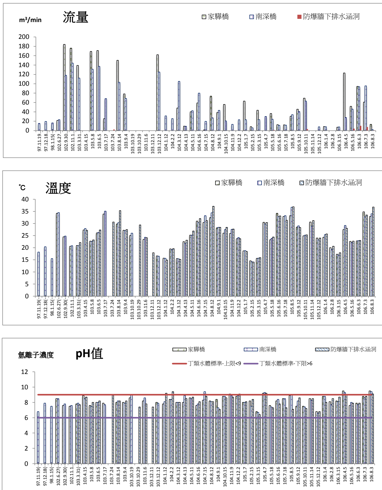
圖 2.4-2 地面水質監測結果圖
