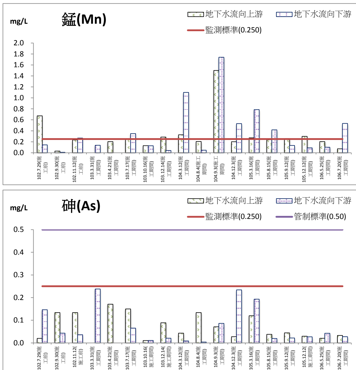
圖 2.5-2 地下水監測結果圖(續)
