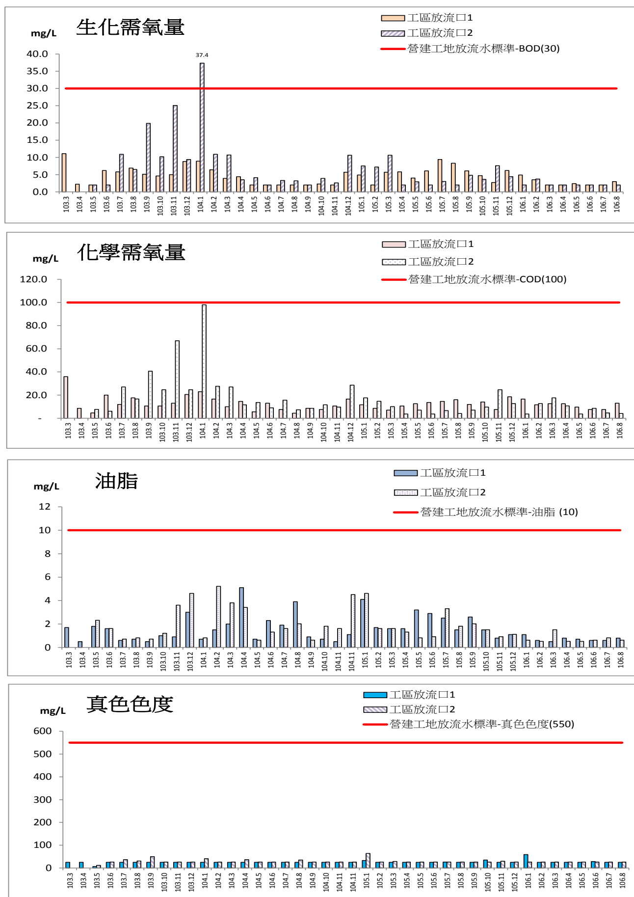
圖 2.6-1 放流水監測結果圖
