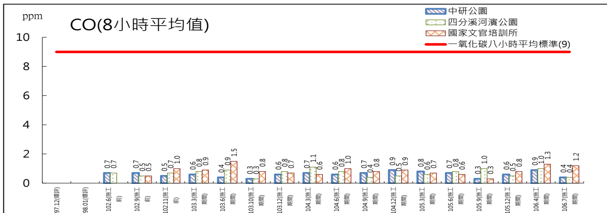
圖 2.1-1 空氣品質監測結果圖(續)
