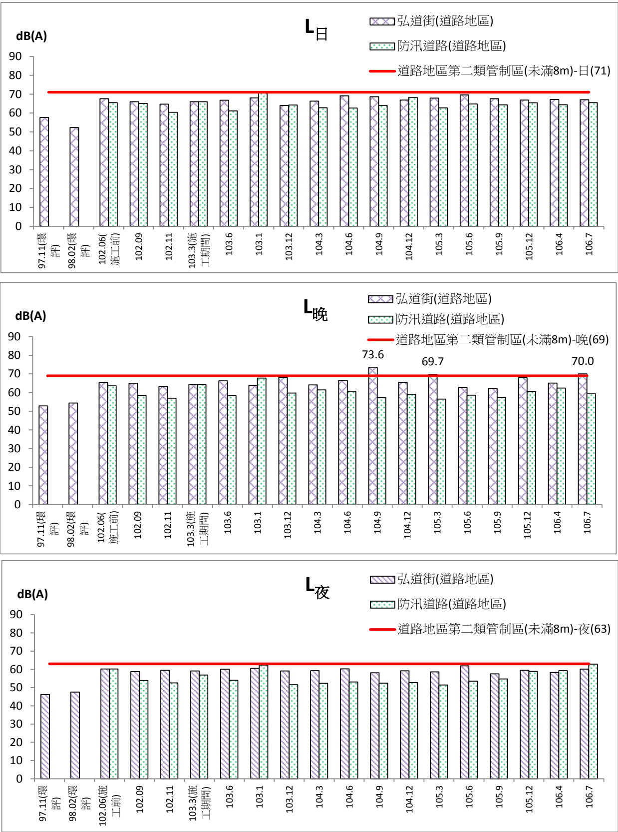
圖 2.2.1-2 弘道街、防汛道路噪音監測結果圖
