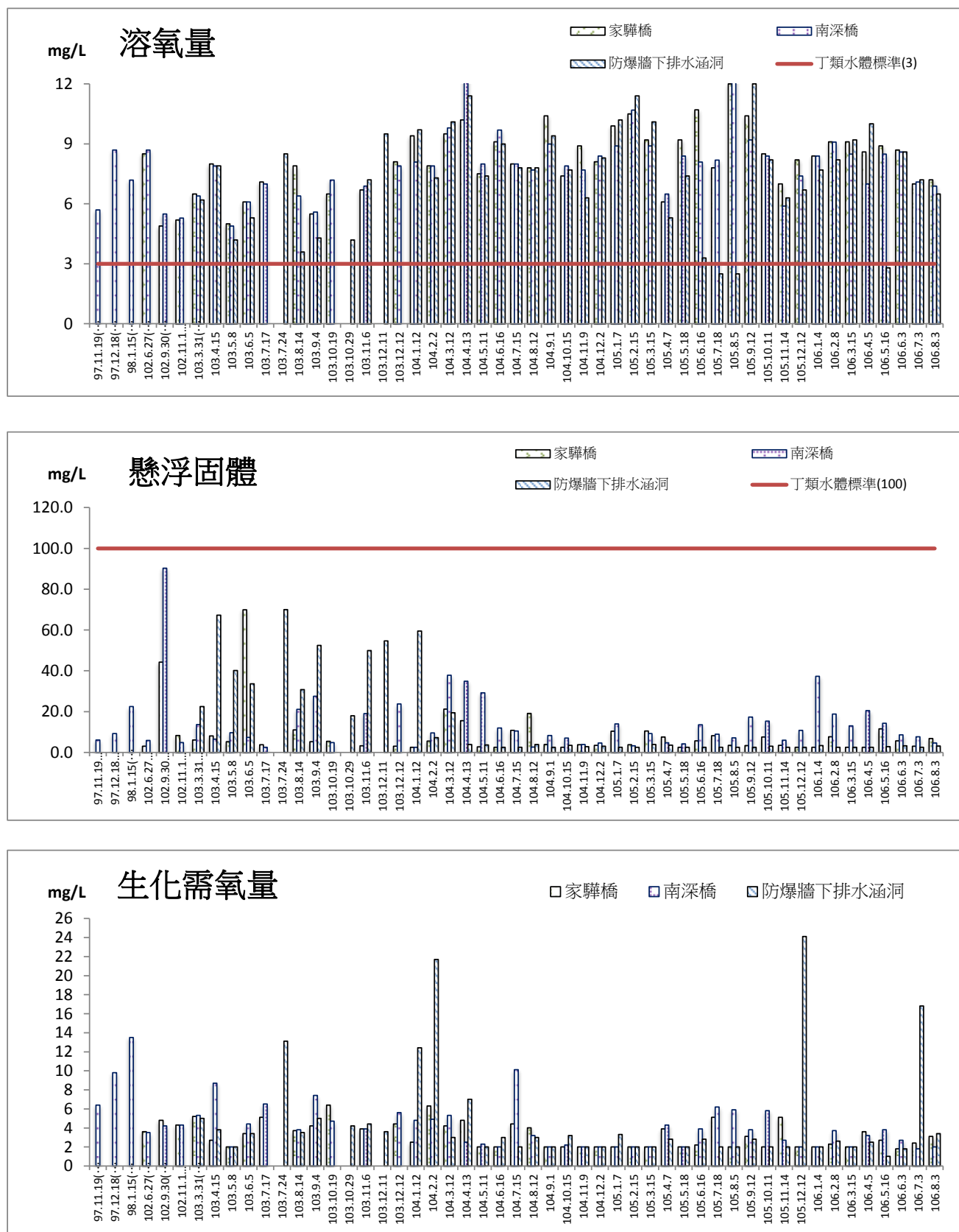
圖 2.4-2 地面水質監測結果圖(續)
