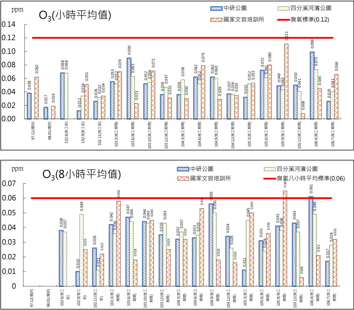
圖 2.1-1 空氣品質監測結果圖(續)
