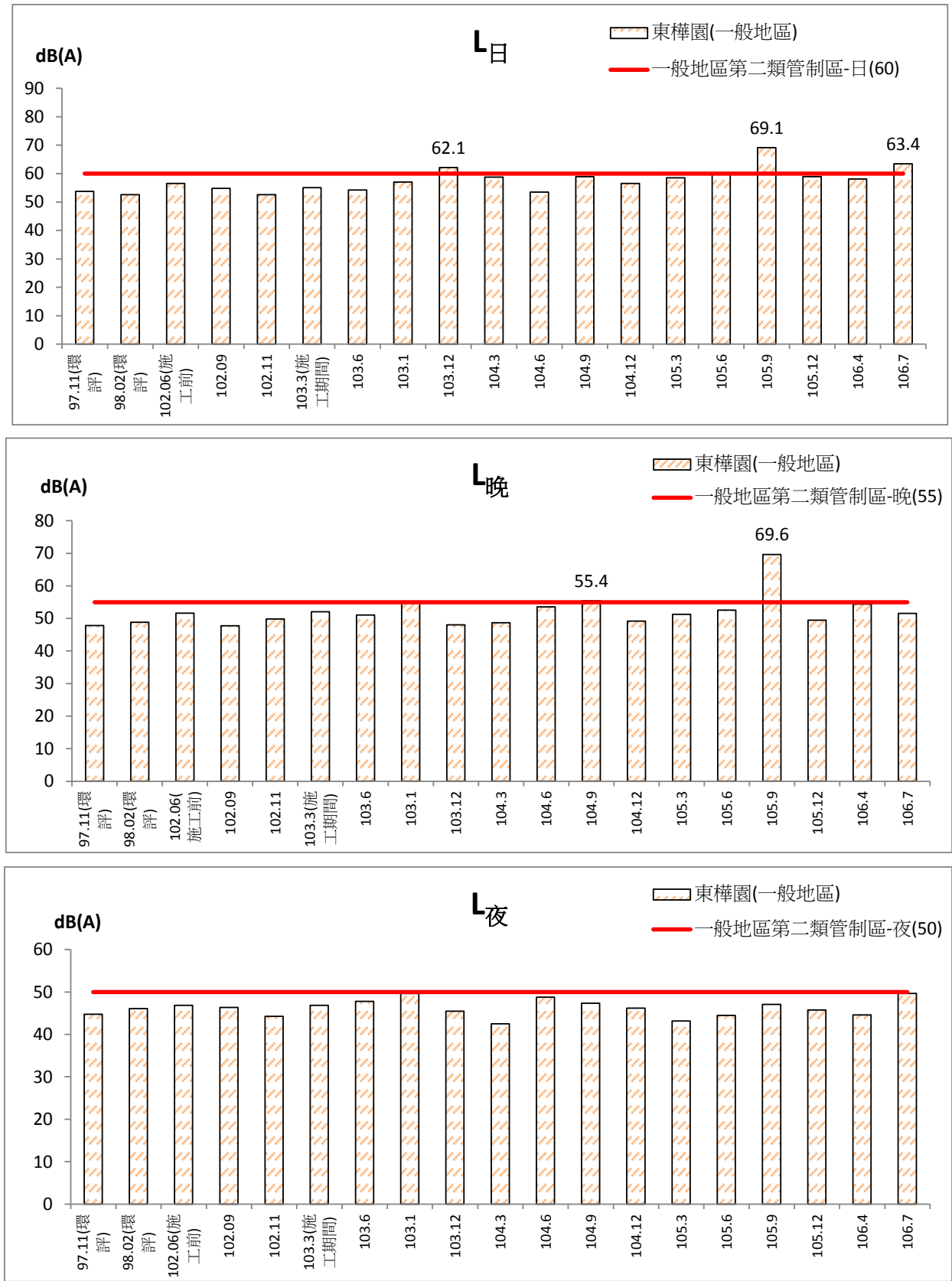
圖 2.2.1-1 東樺園噪音監測結果圖
