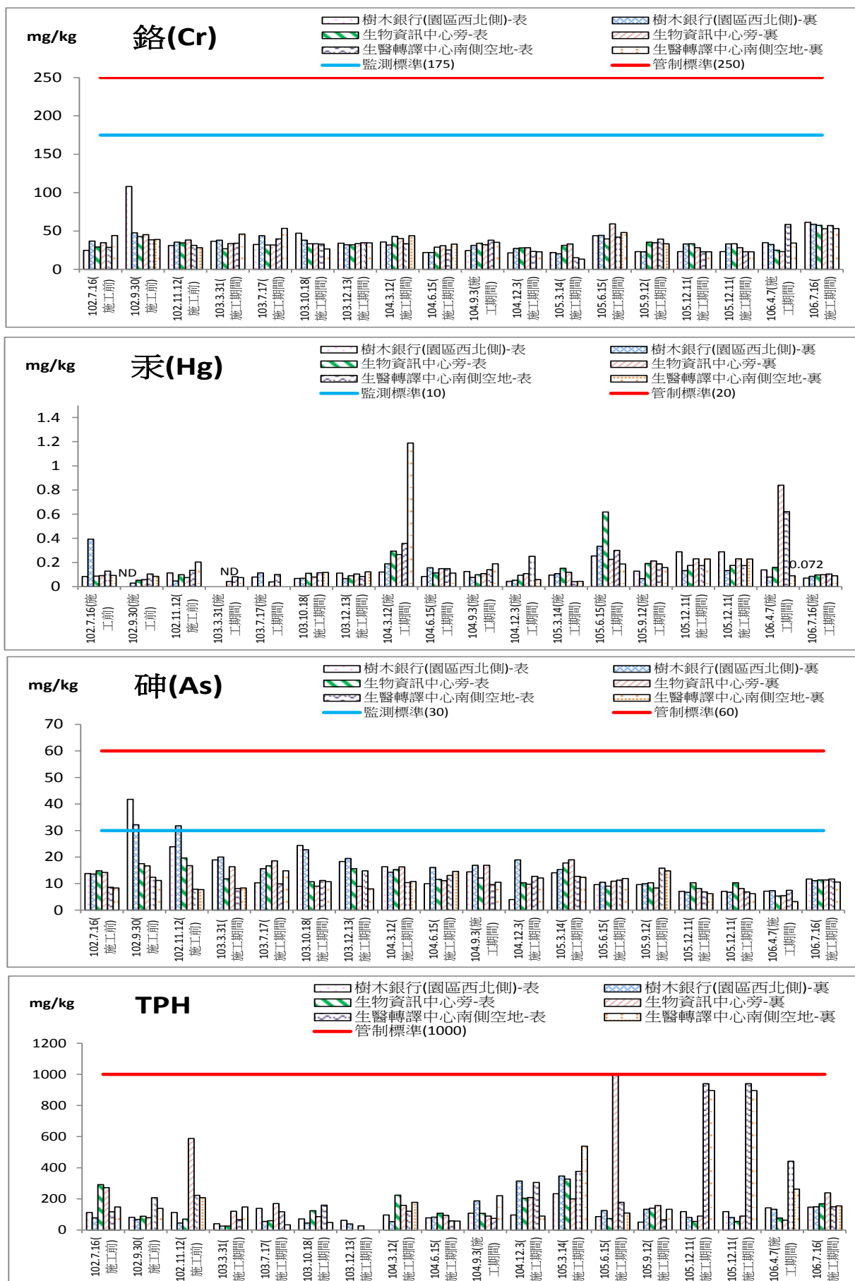
圖 2.3-1 土壤監測結果圖(續)
