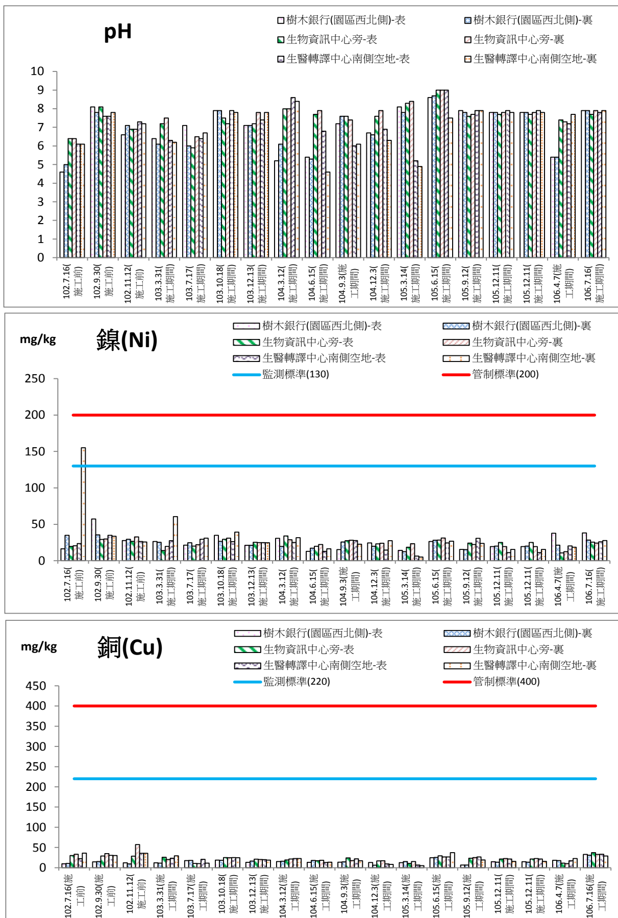
圖 2.3-1 土壤監測結果圖
