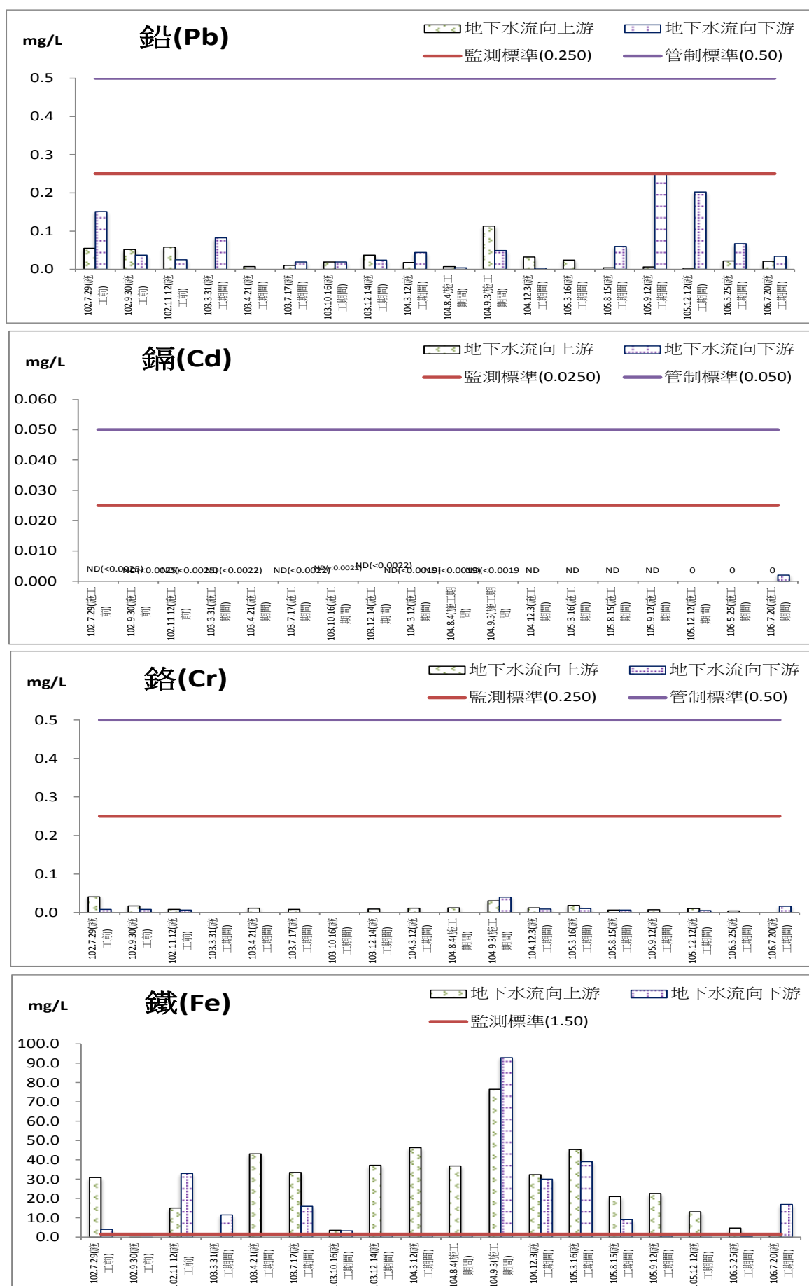
圖 2.5-2 地下水監測結果圖(續)
