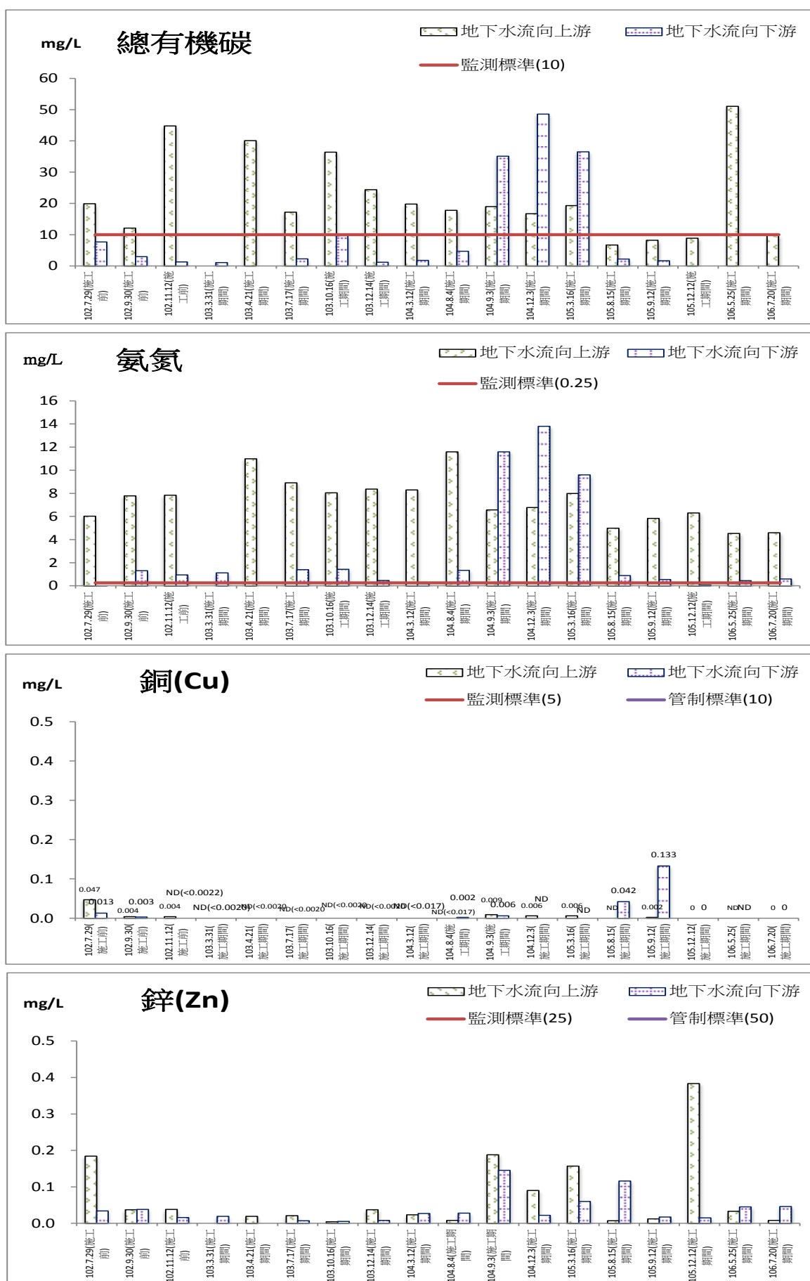
圖 2.5-2 地下水監測結果圖(續)
