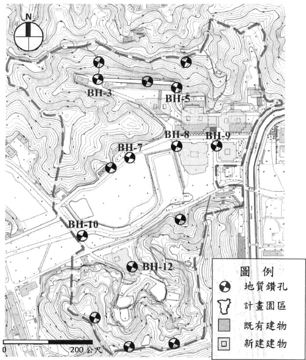
圖 2.5-1 環評階段地下水監測位置圖
