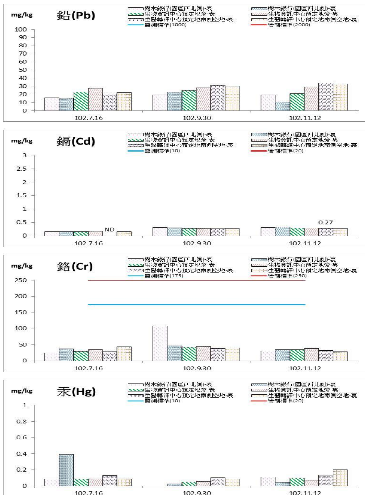
圖 2.3-1 土壤監測結果圖(續)
