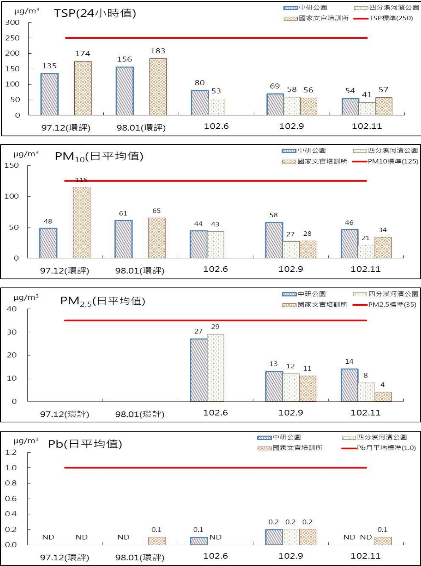
圖 2.1-1 空氣品質監測結果圖
