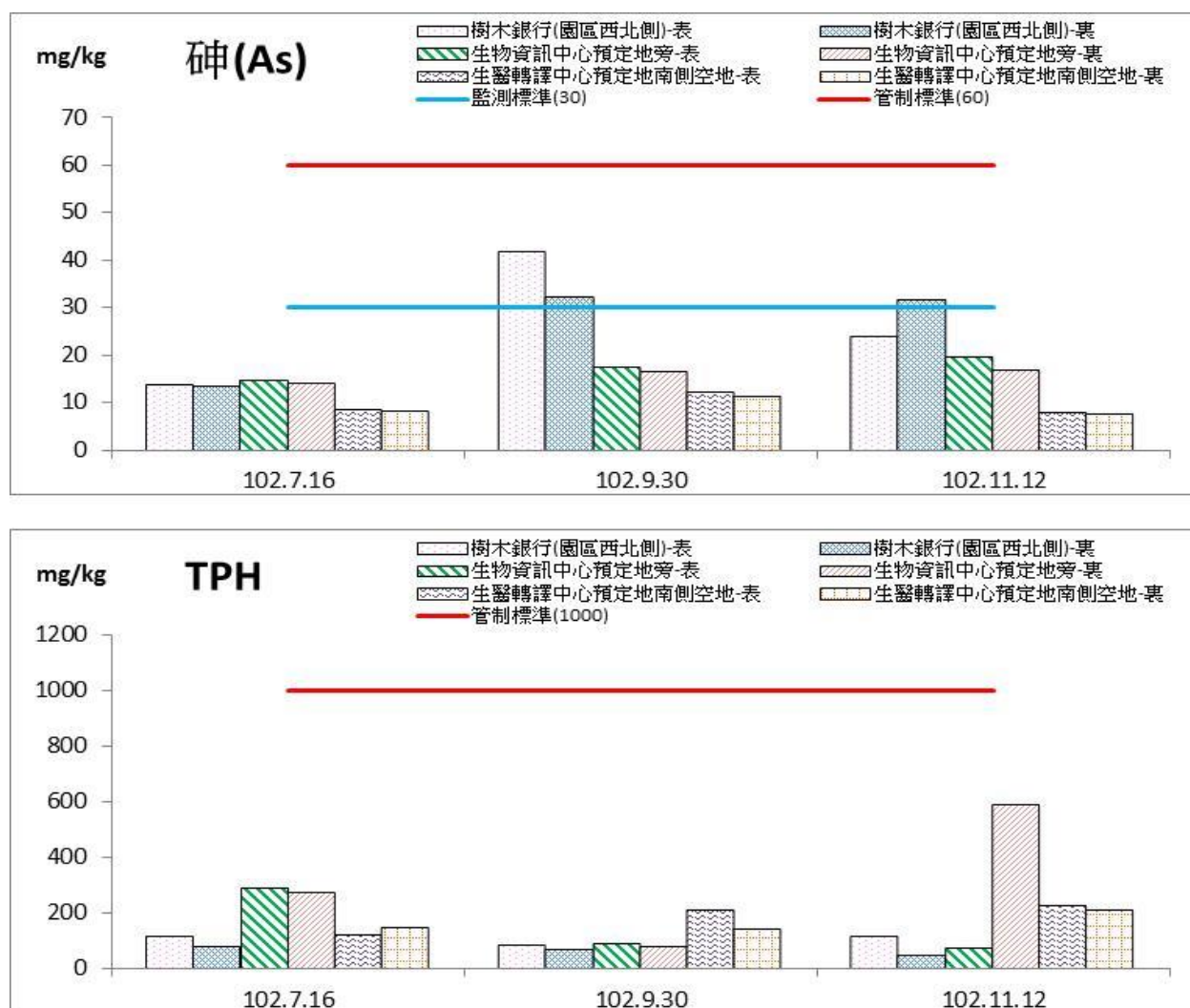
圖 2.3-1 土壤監測結果圖(續)
