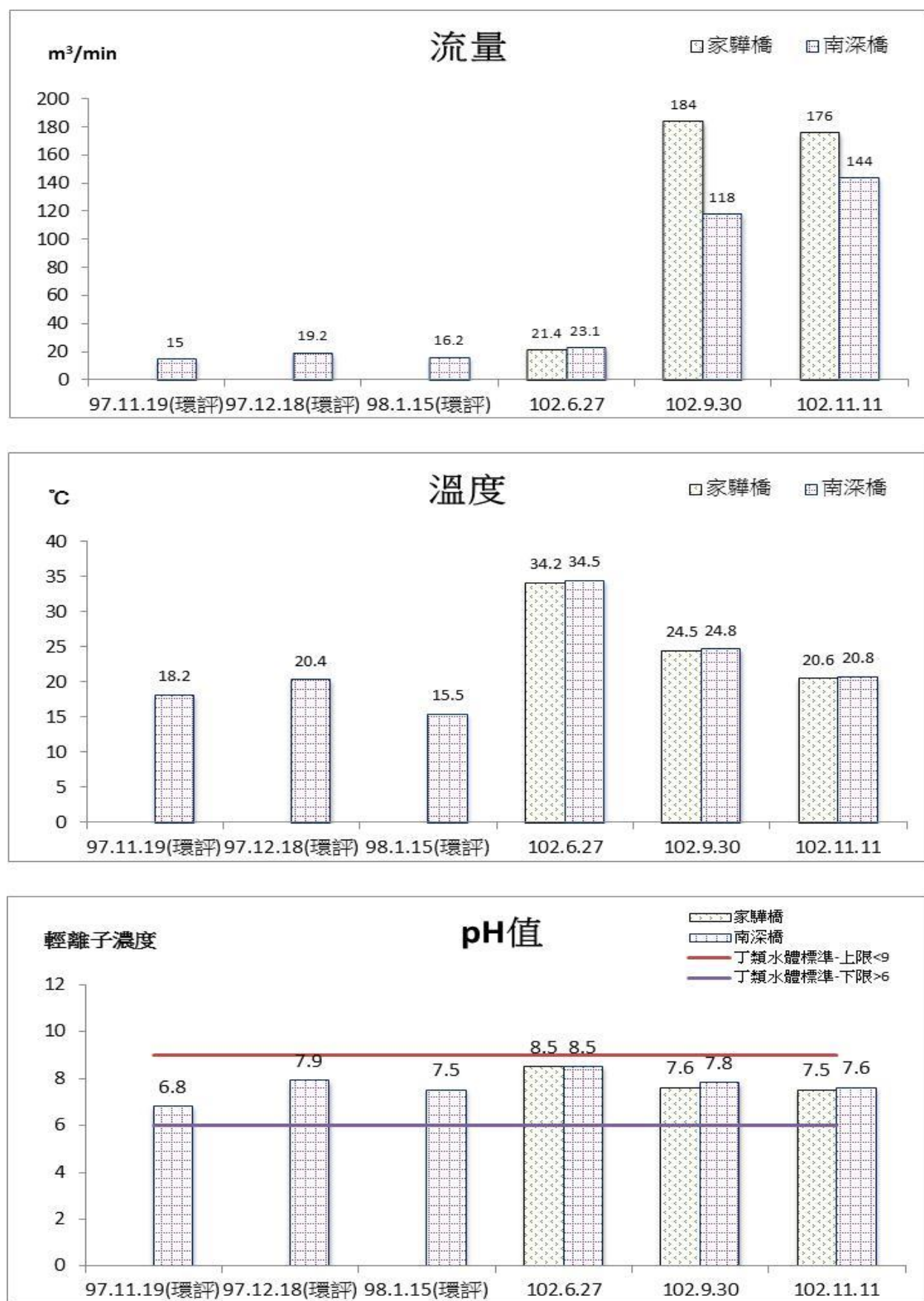
圖 2.4-2 地面水質監測結果圖
