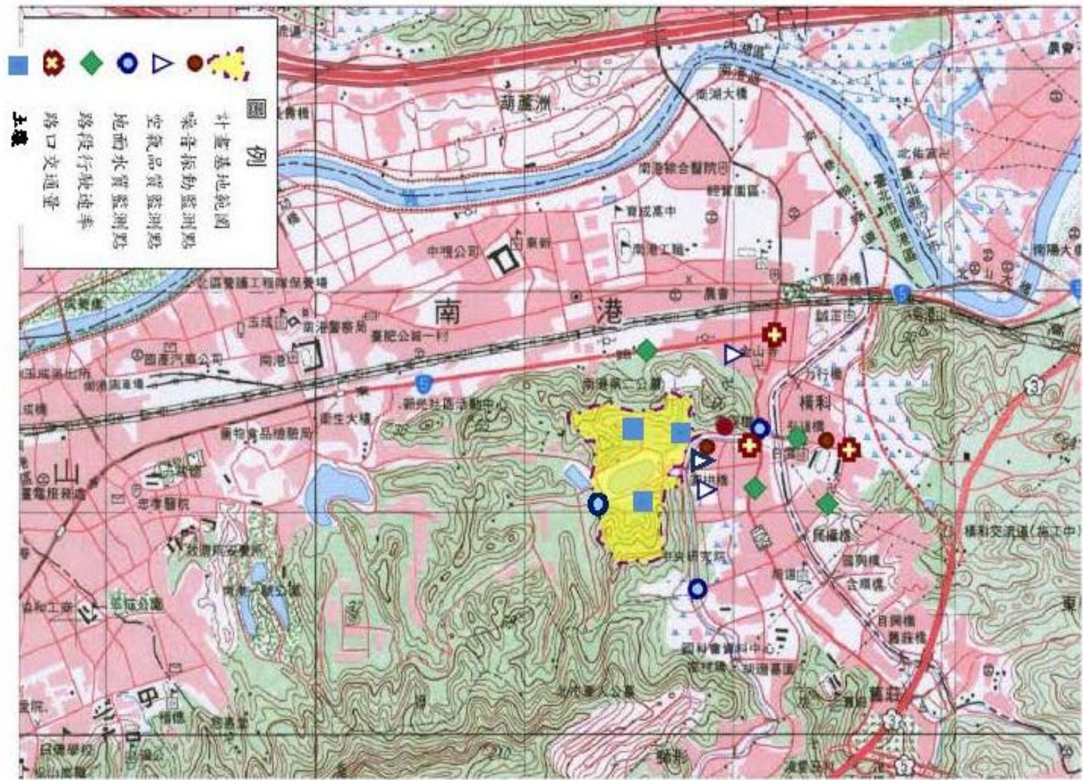
圖 1.4-1 本計畫環境監測位置示意圖
