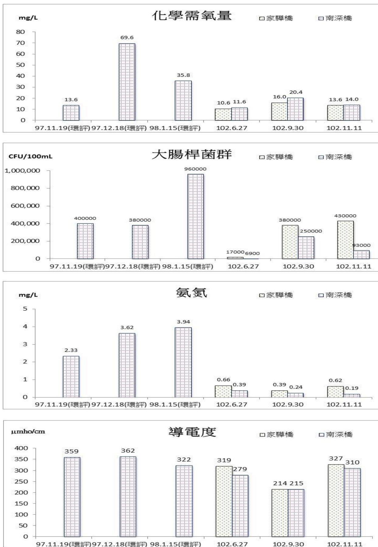
圖 2.4-2 地面水質監測結果圖(續)
