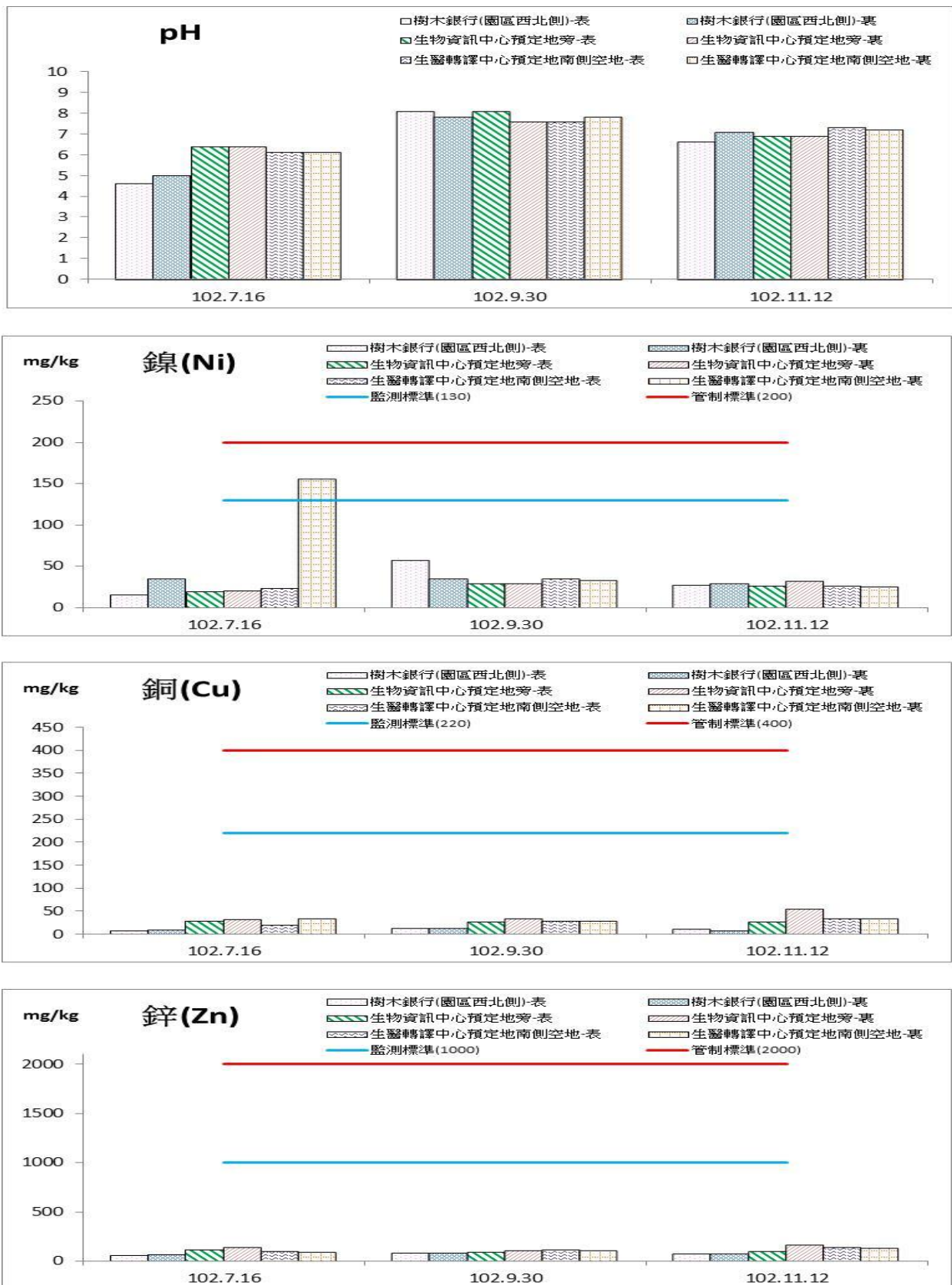
圖 2.3-1 土壤監測結果圖
