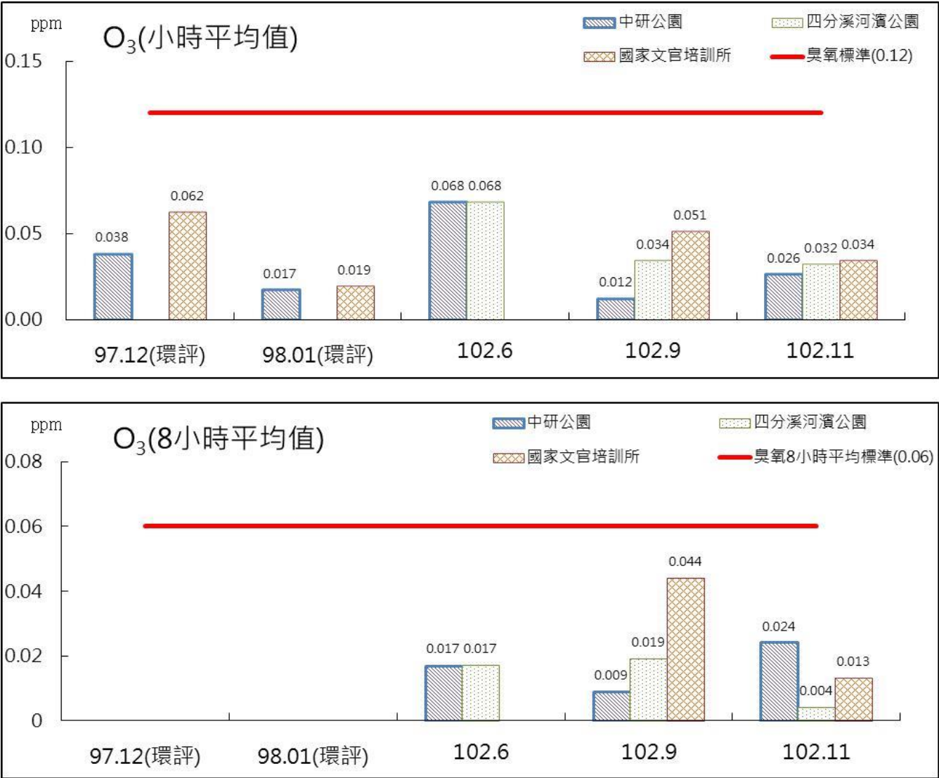
圖 2.1-1 空氣品質監測結果圖(續)
