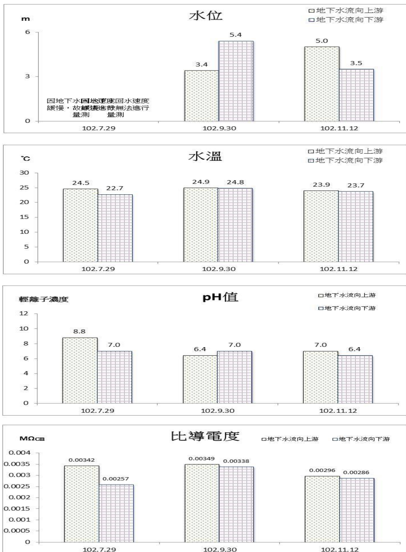
圖 2.5-2 地下水監測結果圖
