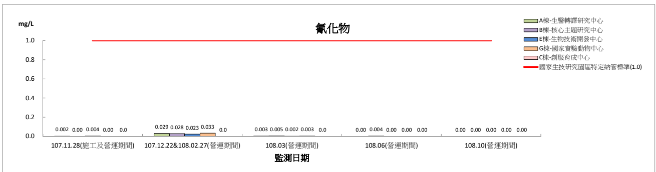
圖 2.8-1 實驗室廢水納管水質監測結果圖(營運期間)(續 5)
