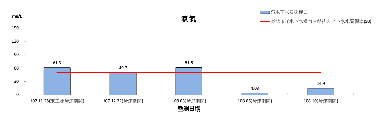
圖 2.7-1 園區污水納管水質監測結果圖(營運期間)(續 6)
