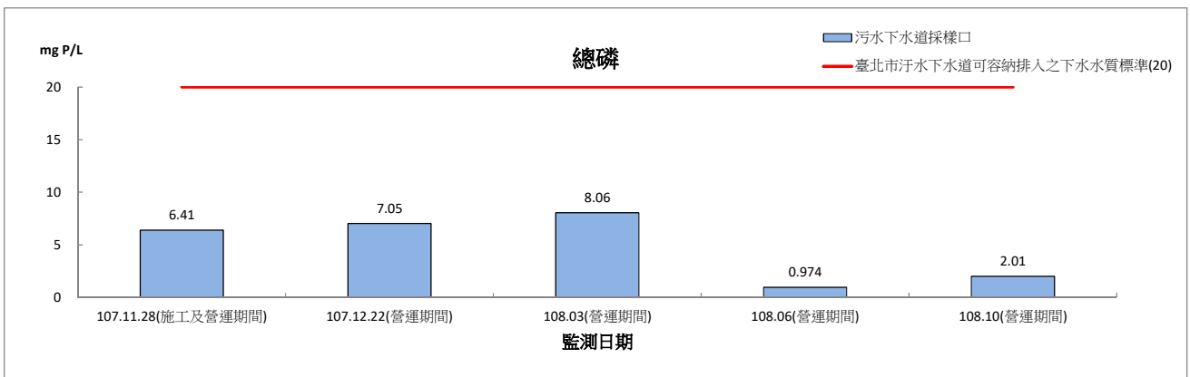
圖 2.7-1 園區污水納管水質監測結果圖(營運期間)(續 2)
