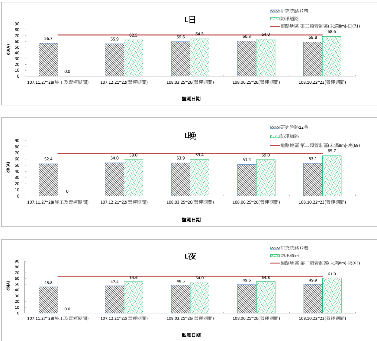
圖 2.2.1-4 研究院路 12 巷、防汛道路噪音監測結果圖(營運期間)
