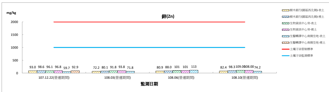
圖 2.3-2 土壤監測結果圖(營運期間)
