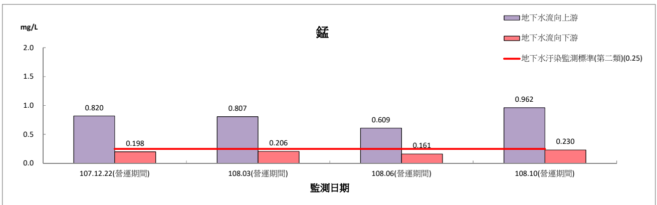
圖 2.5-3 地下水監測結果圖(營運期間)(續 3)
