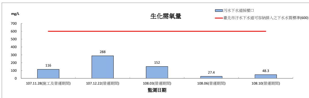
圖 2.7-1 園區污水納管水質監測結果圖(營運期間)
