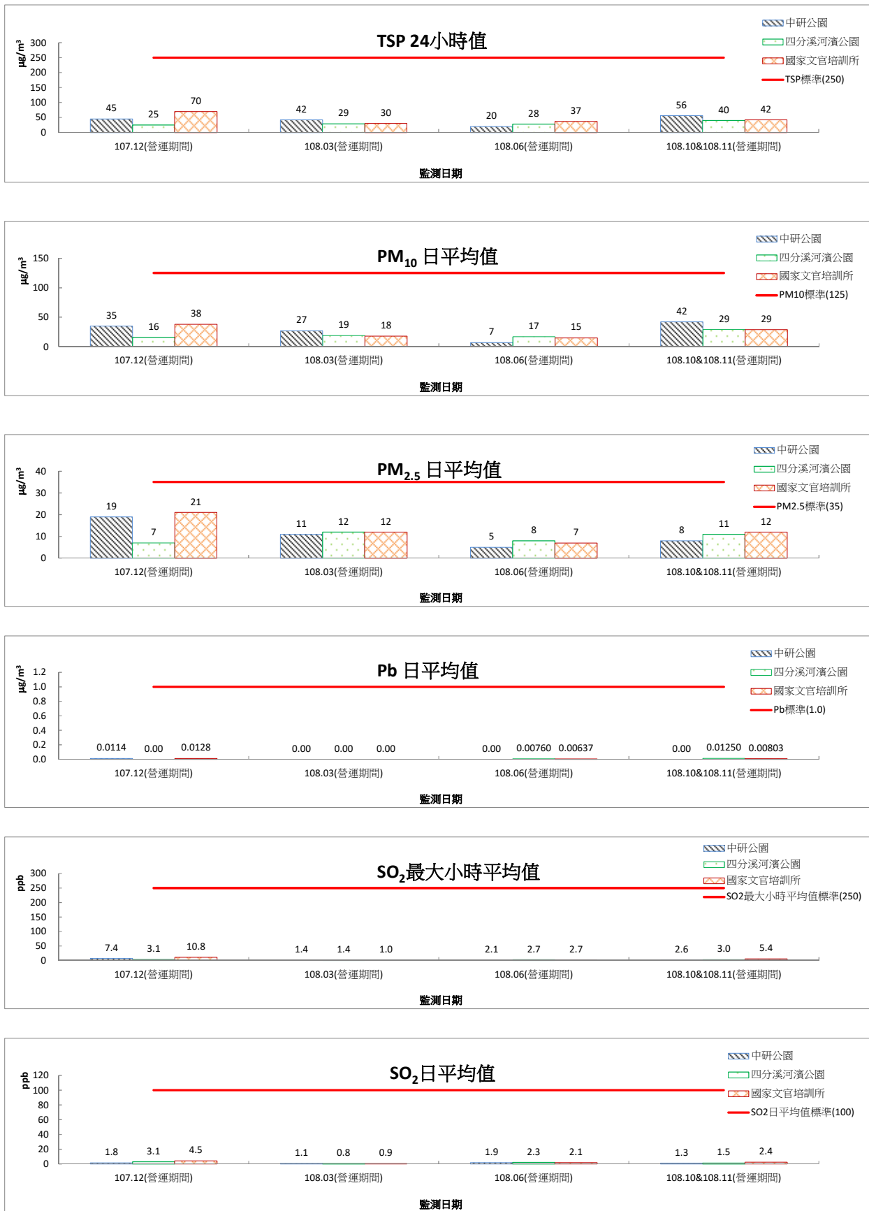
圖 2.1-2 空氣品質監測結果圖(營運期間)
