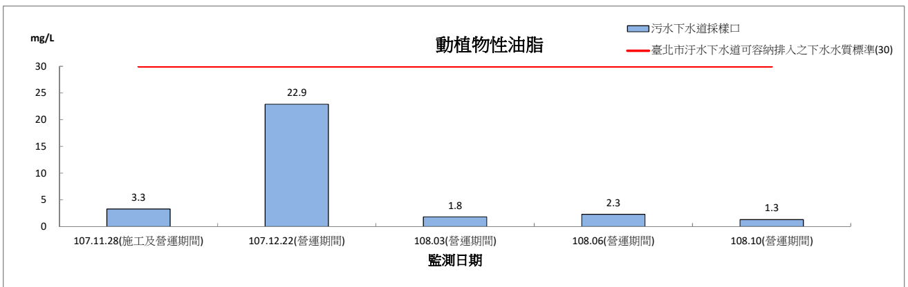
圖 2.7-1 園區污水納管水質監測結果圖(營運期間)(續 1)
