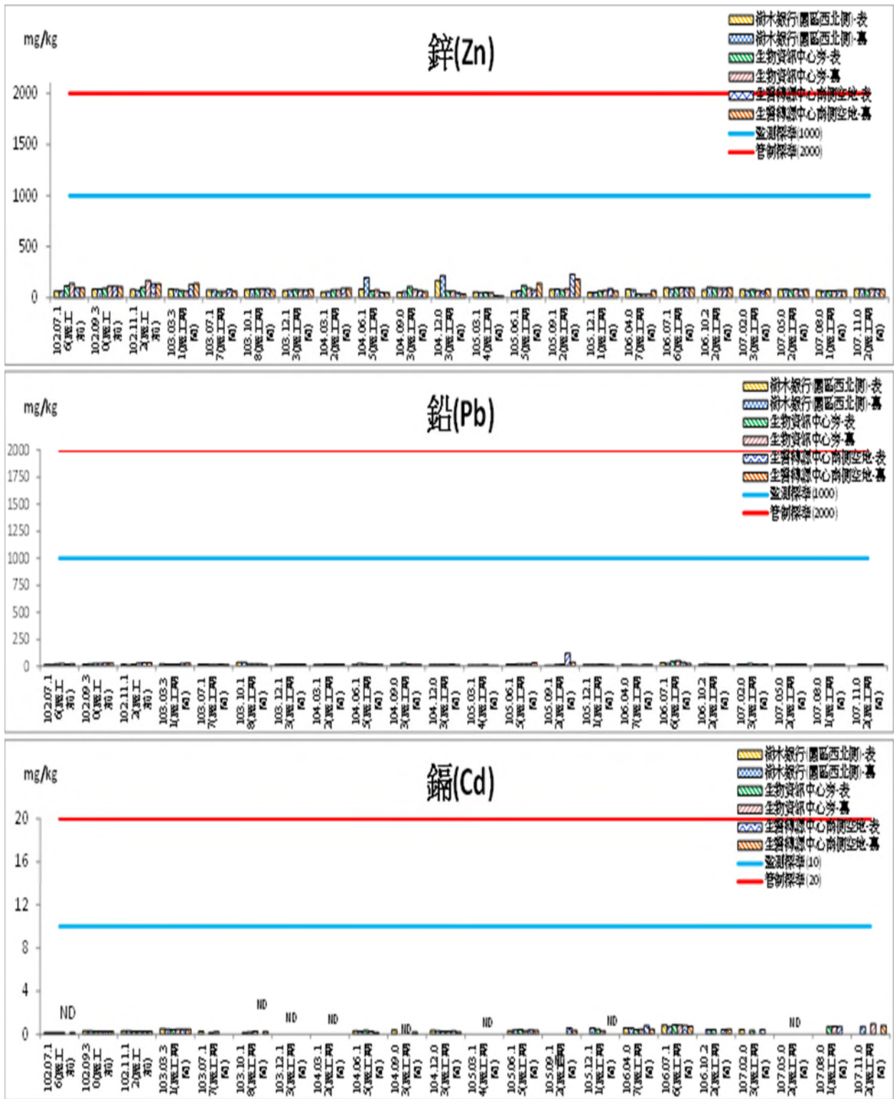
圖 2.3-1 土壤監測結果圖(施工期間)(續 1)
