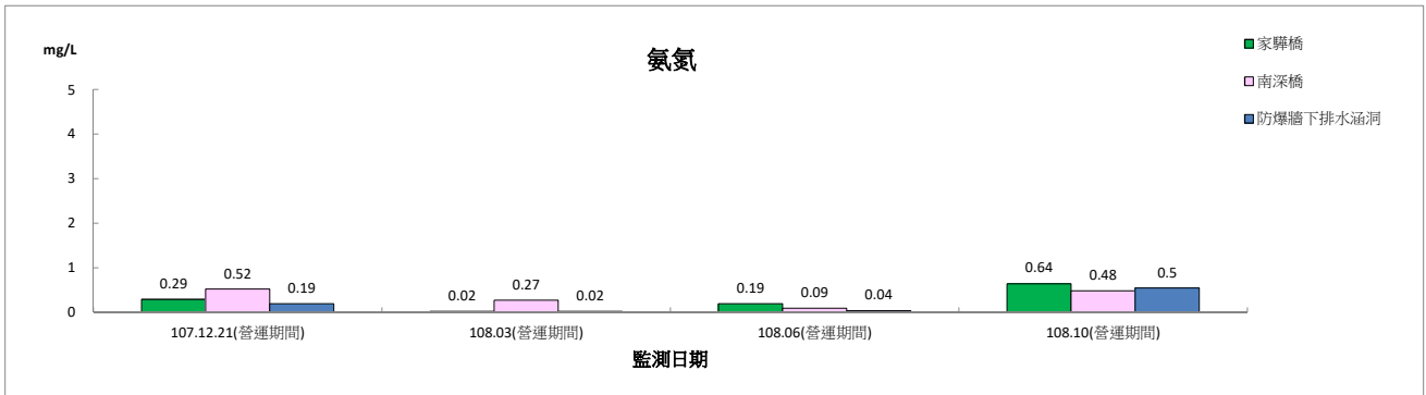
圖 2.4-3 地面水質監測結果圖(營運期間)(續 2)
