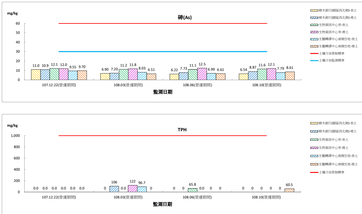
圖 2.3-2 土壤監測結果圖(營運期間)(續 2)
