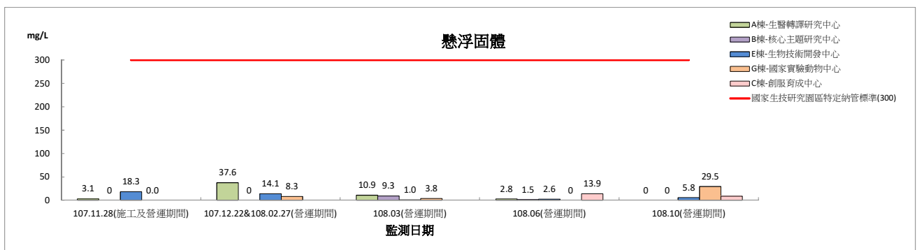
圖 2.8-1 實驗室廢水納管水質監測結果圖(營運期間)
