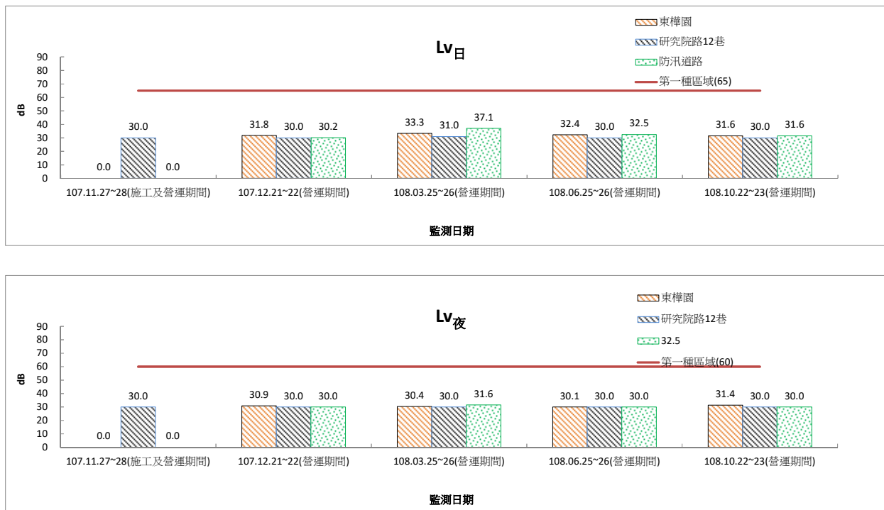
圖 2.2.2-2 振動監測結果圖(營運期間)
