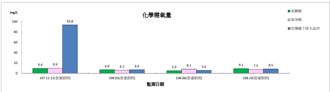
圖 2.4-3 地面水質監測結果圖(營運期間)(續 1)
