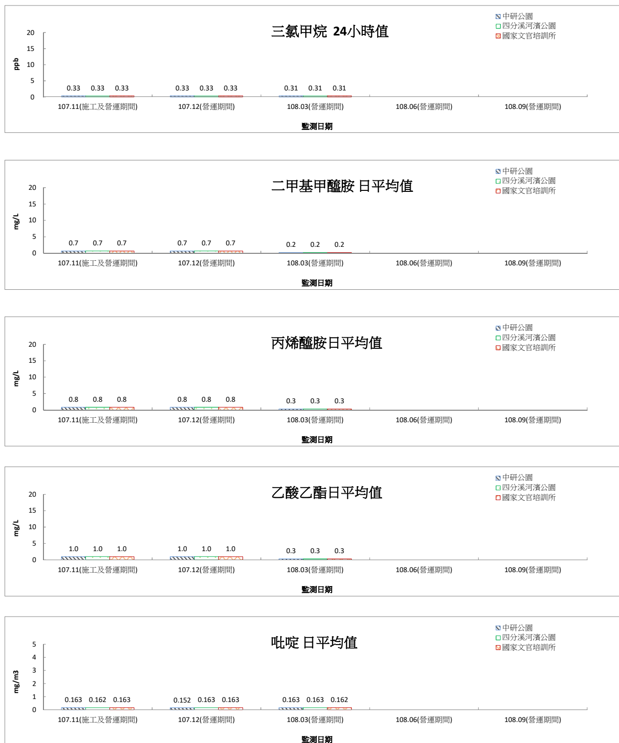
圖 2.1-2 空氣品質監測結果圖(營運期間)(續 3)
