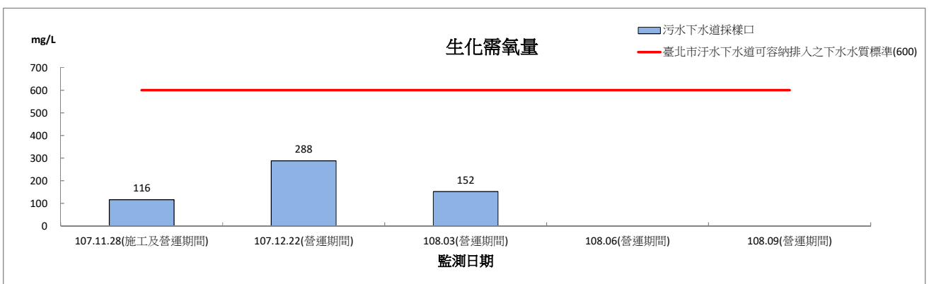
圖 2.7-1 園區污水納管水質監測結果圖(營運期間)
