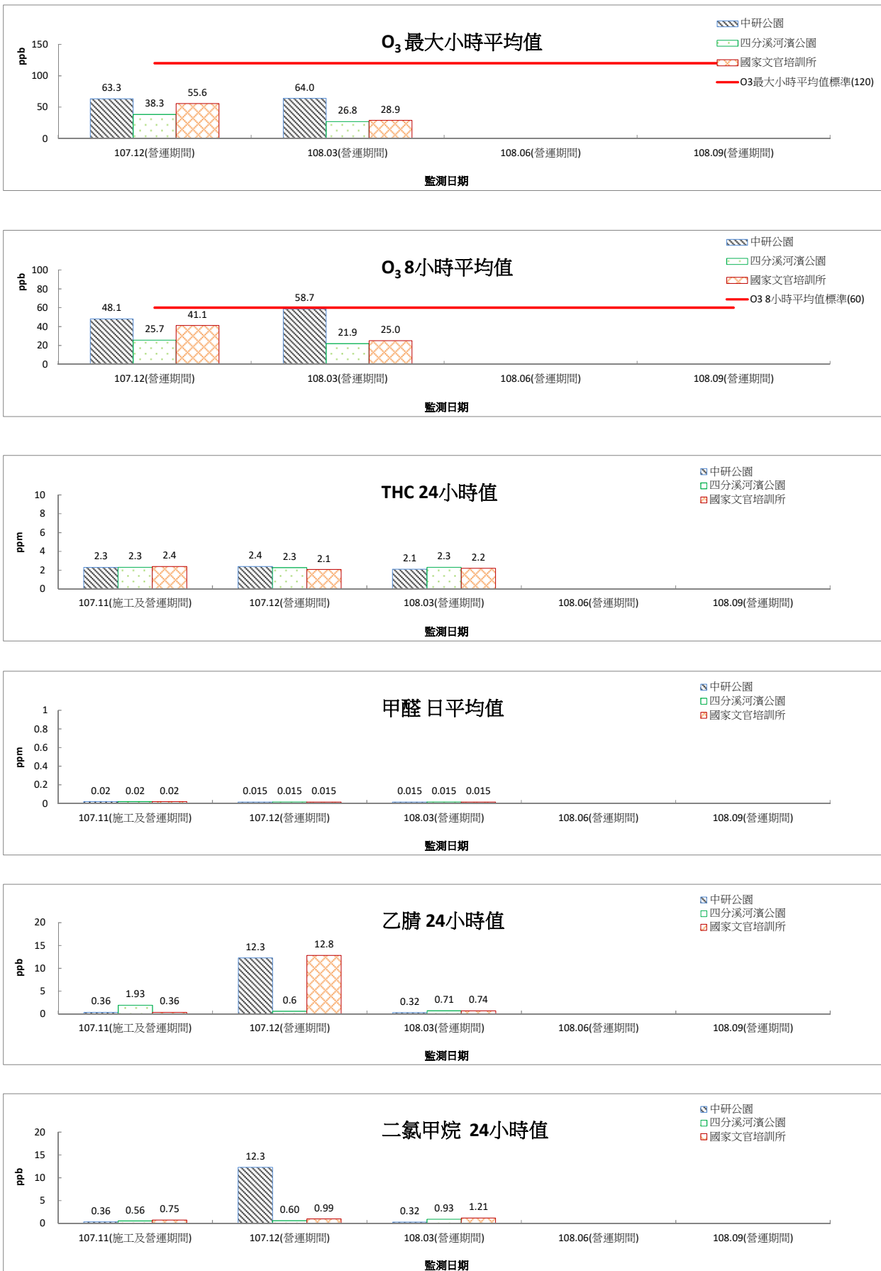
圖 2.1-2 空氣品質監測結果圖(營運期間)(續 2)
