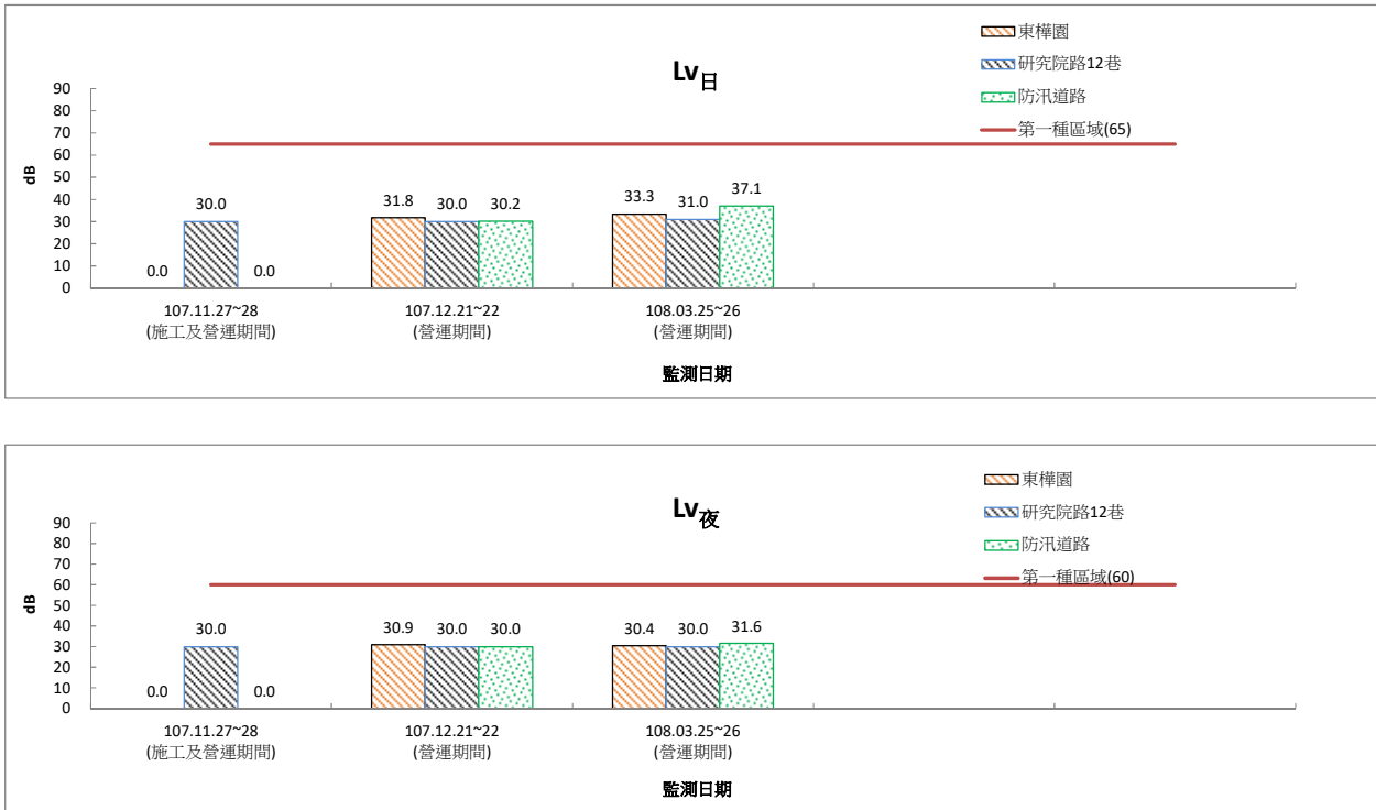
圖 2.2.2-2 振動監測結果圖(營運期間)
