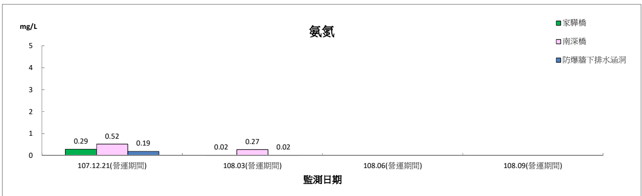
圖 2.4-3 地面水質監測結果圖(營運期間)(續 2)
