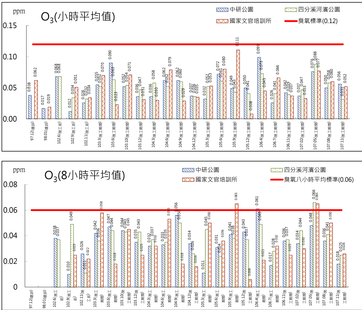
圖 2.1-1 空氣品質監測結果(施工期間)(續 3)
