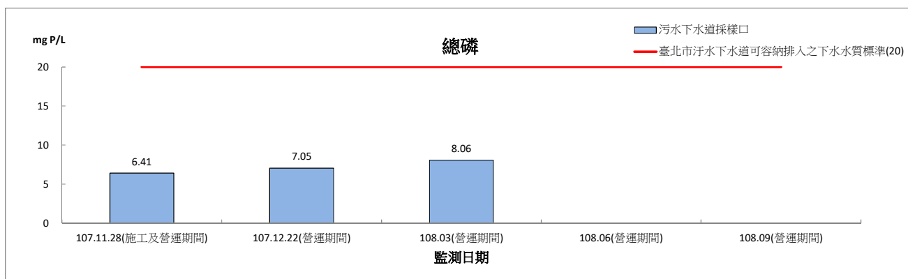
圖 2.7-1 園區污水納管水質監測結果圖(營運期間)(續 2)
