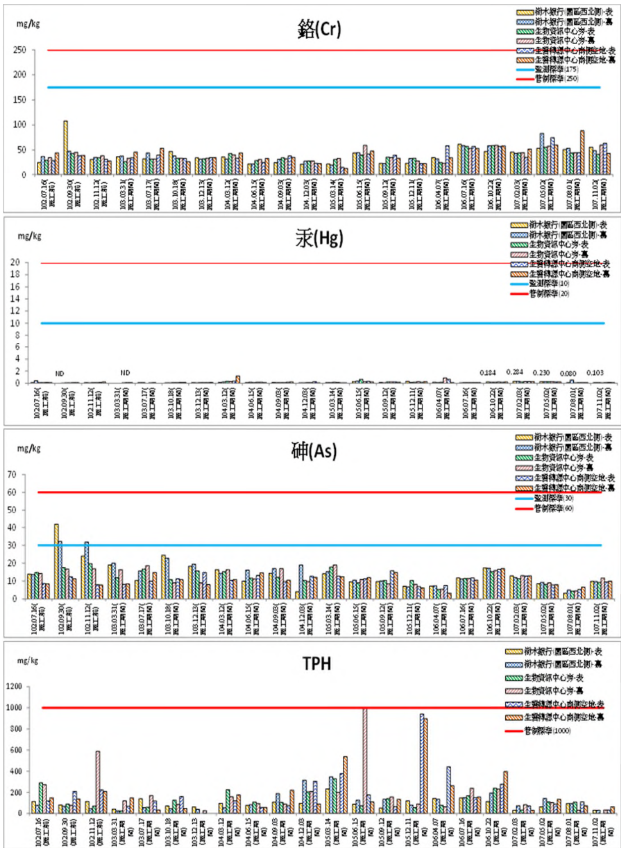
圖 2.3-1 土壤監測結果圖(施工期間)(續 2)
