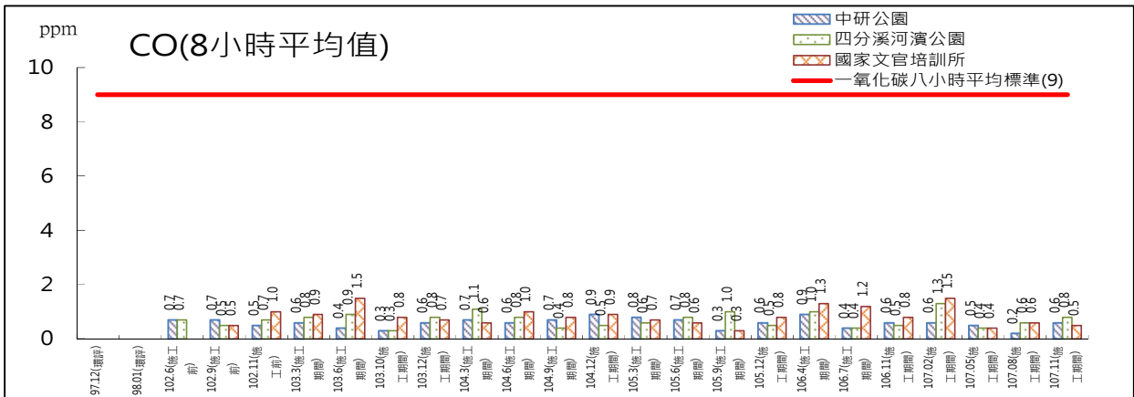
圖 2.1-1 空氣品質監測結果圖(施工期間)(續 2)
