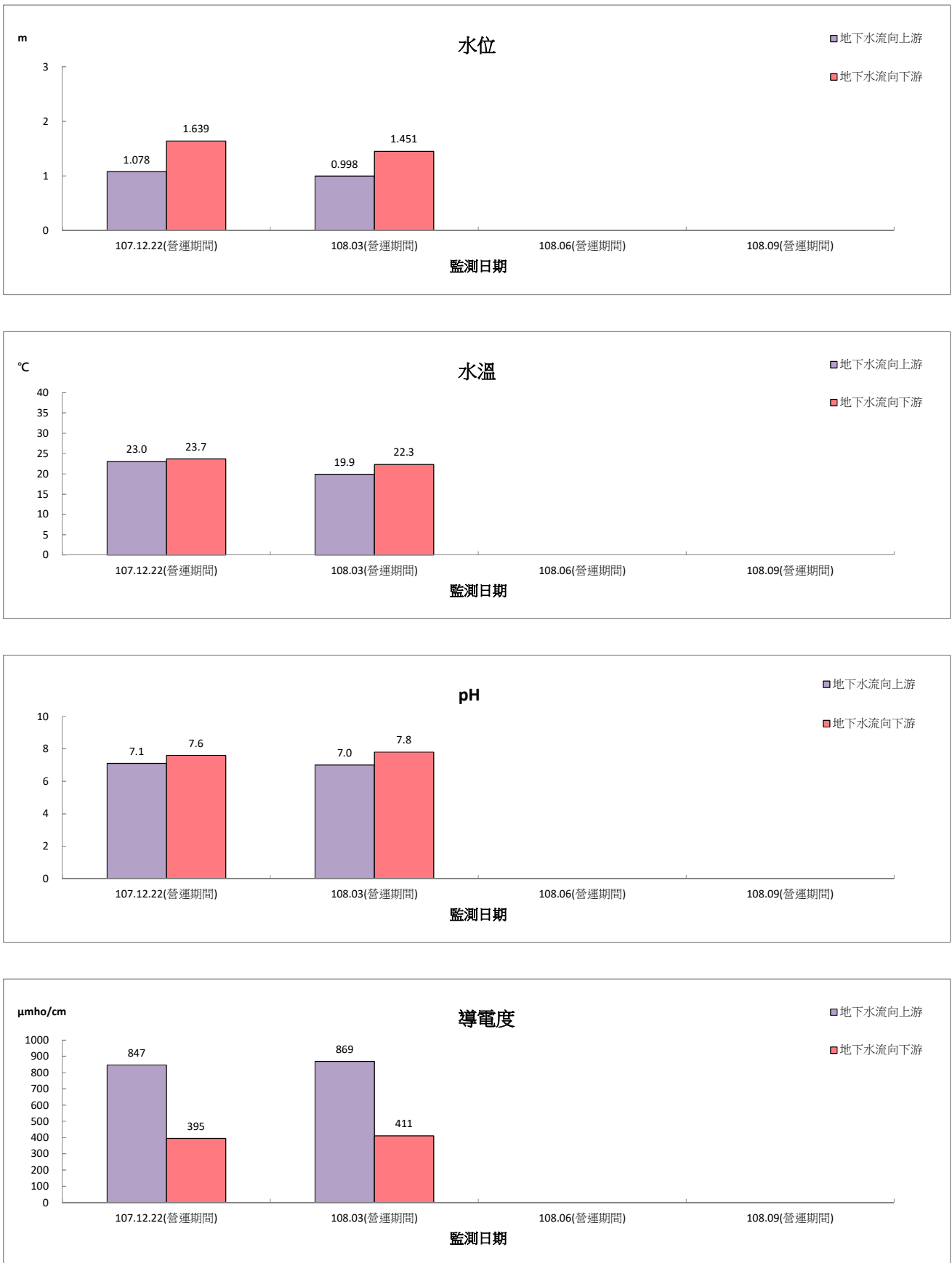
圖 2.5-3 地下水監測結果圖(營運期間)
