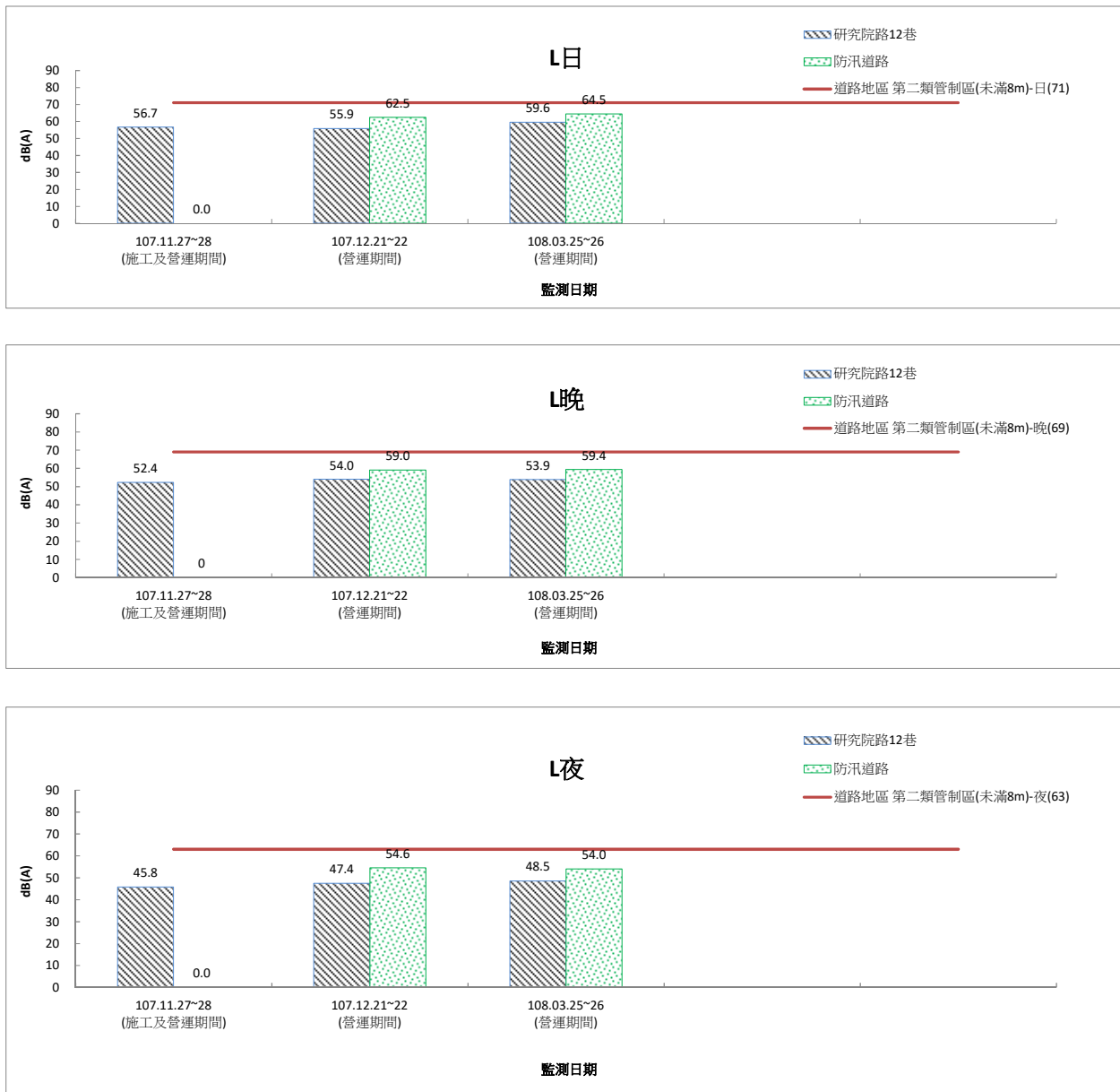
圖 2.2.1-4 研究院路 12 巷、防汛道路噪音監測結果圖(營運期間)
