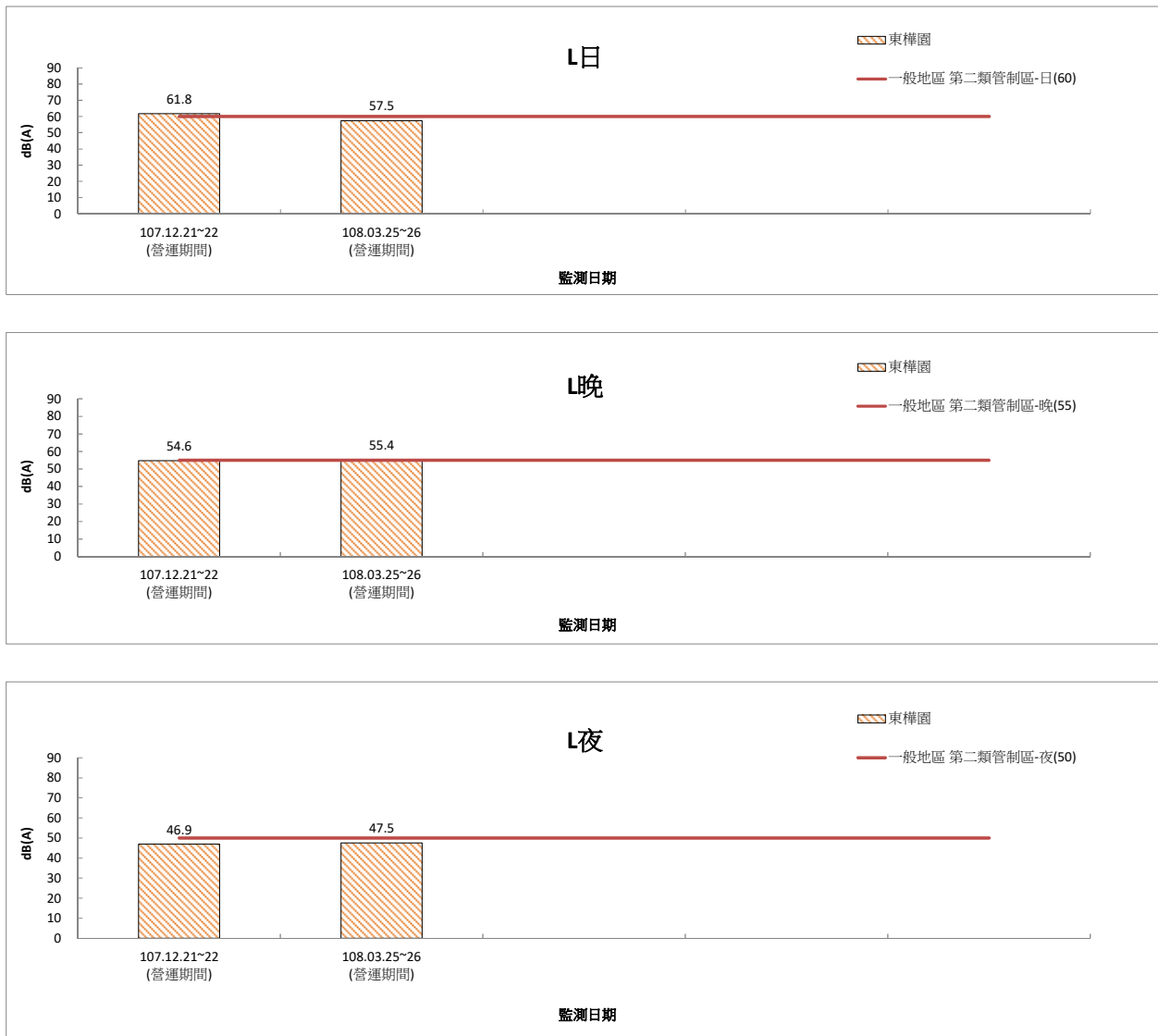
圖 2.2.1-2 東樺園噪音監測結果圖(營運期間)
