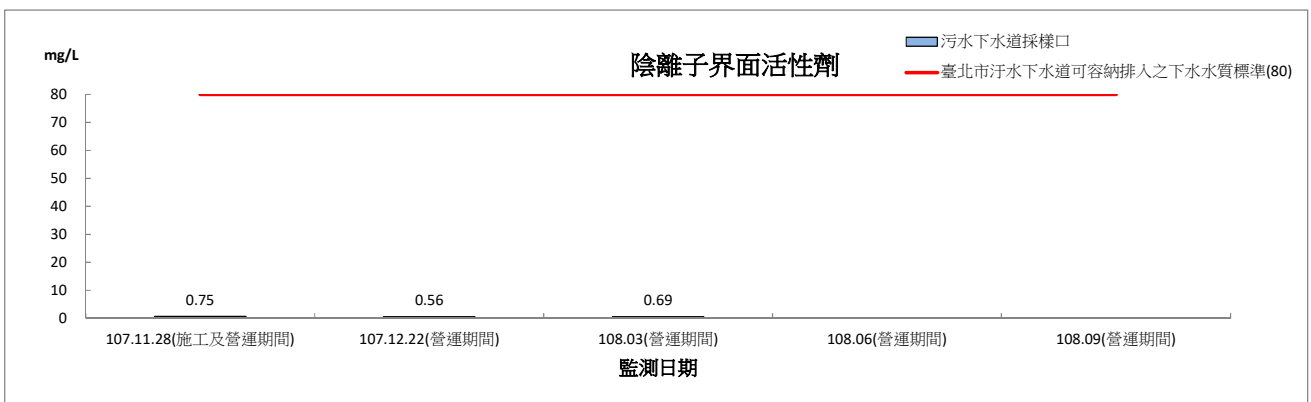
圖 2.7-1 園區污水納管水質監測結果圖(營運期間)(續 5)
