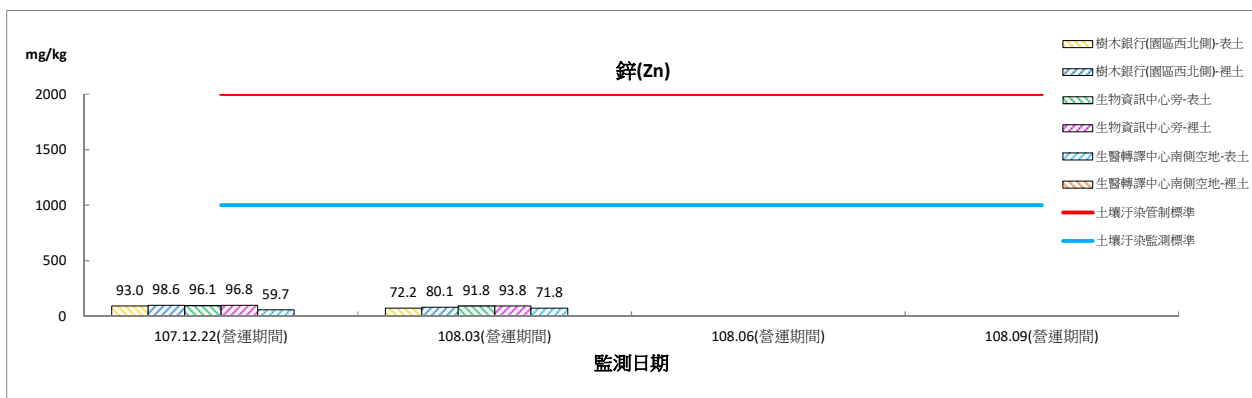
圖 2.3-2 土壤監測結果圖(營運期間)
