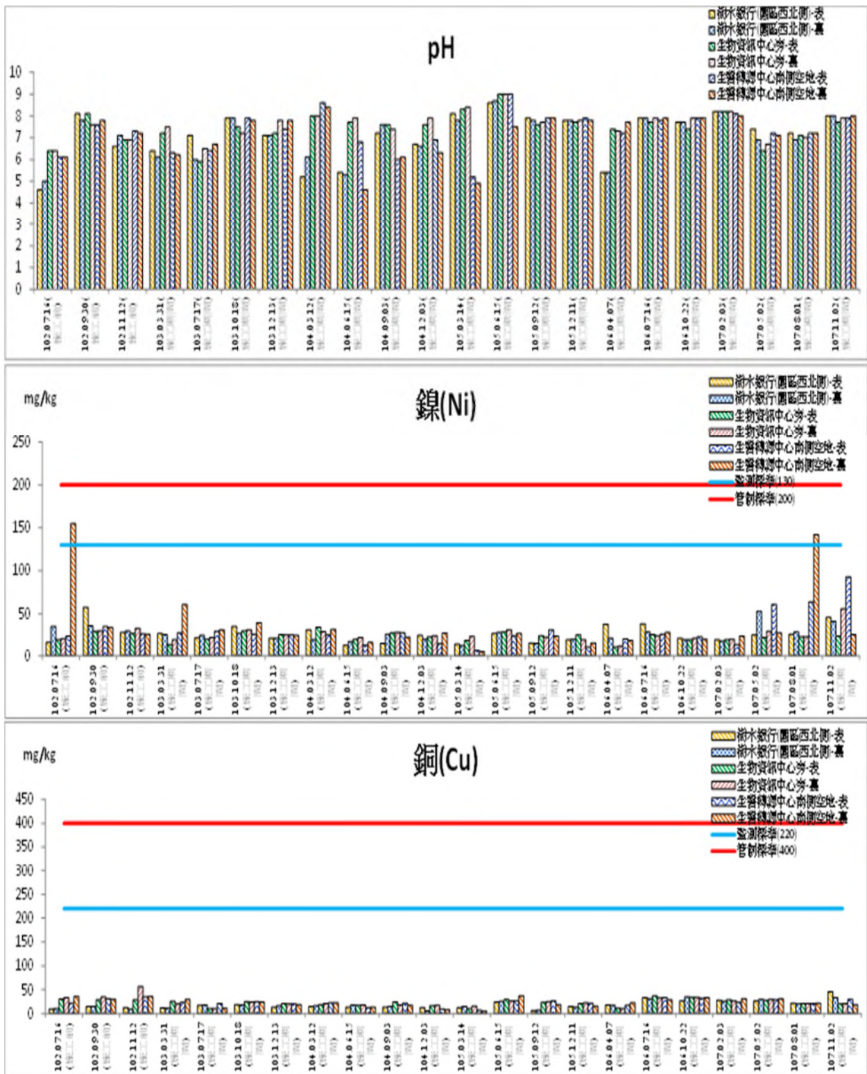
圖 2.3-1 土壤監測結果圖(施工期間)
