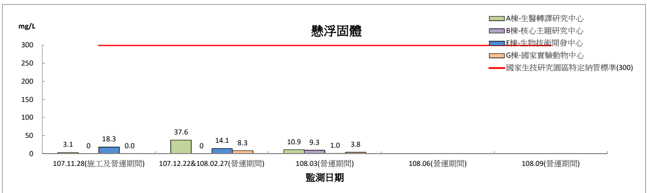
圖 2.8-1 實驗室廢水納管水質監測結果圖(營運期間)
