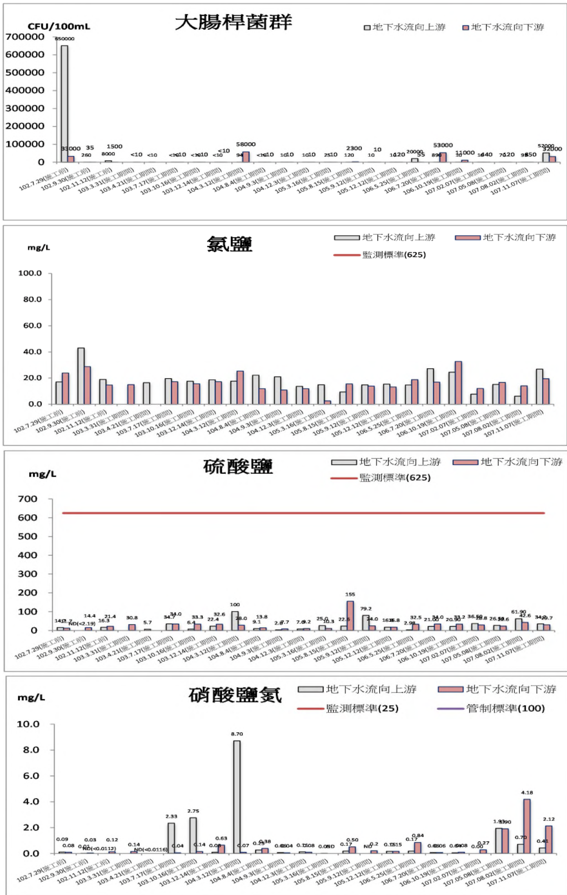
圖 2.5-2 地下水監測結果圖(施工期間)(續 1)
