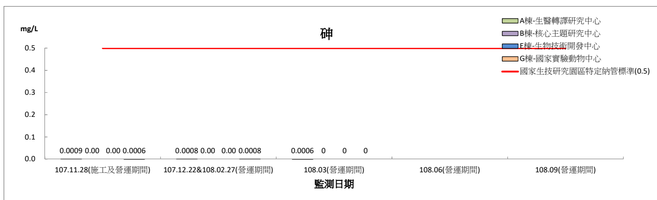
圖 2.8-1 實驗室廢水納管水質監測結果圖(營運期間)(續 2)
