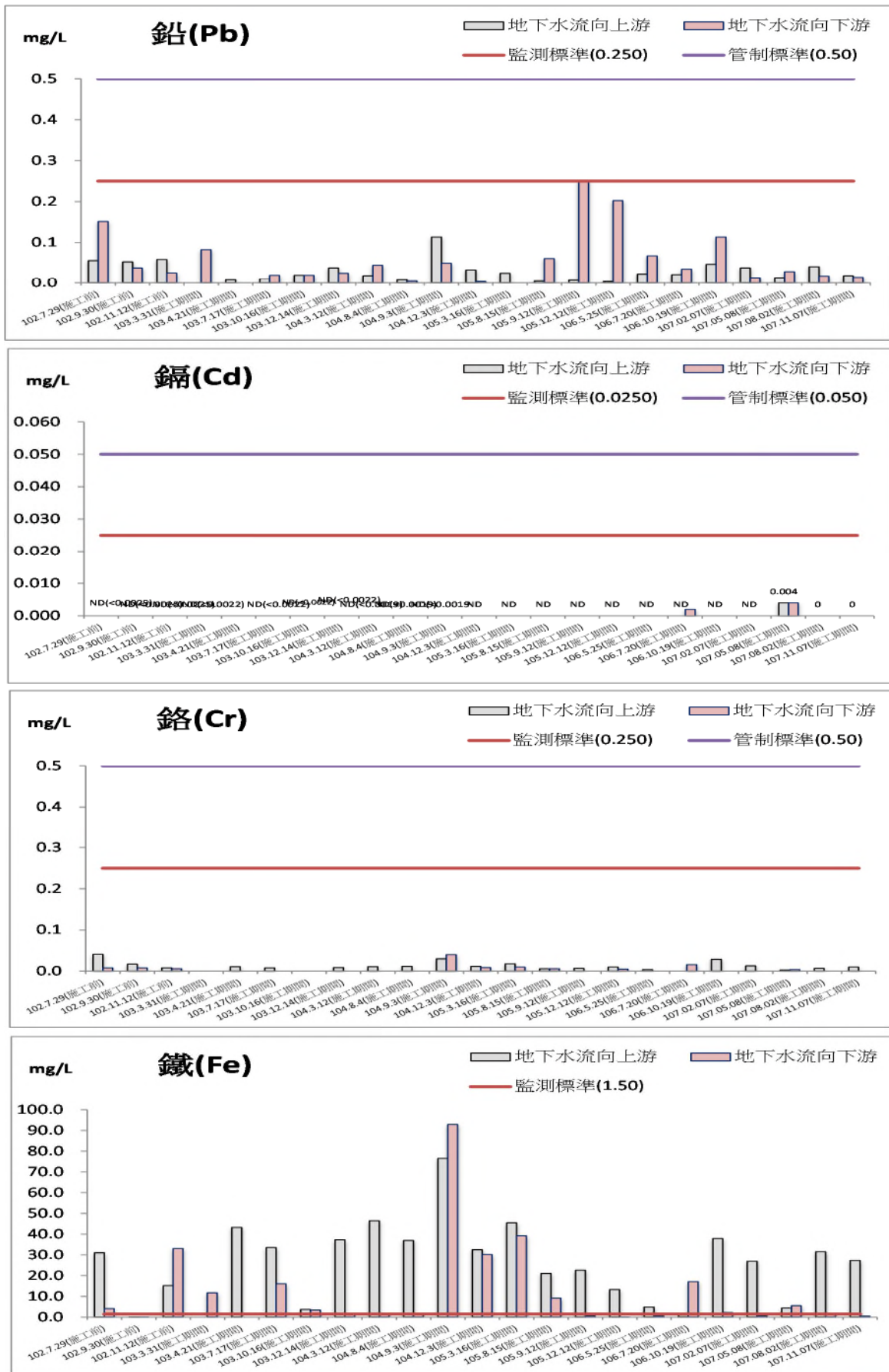
圖 2.5-2 地下水監測結果圖(施工期間)(續 3)
