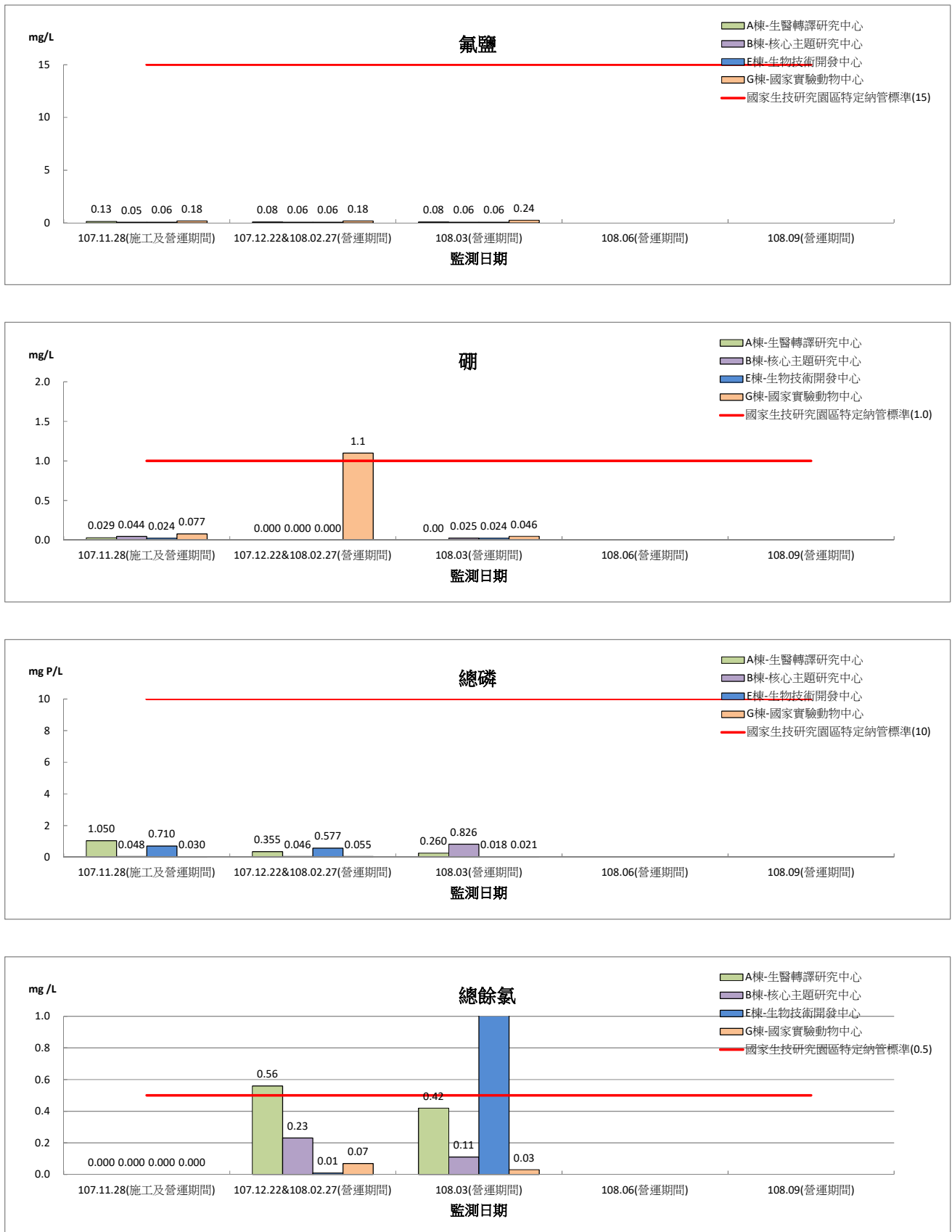
圖 2.8-1 實驗室廢水納管水質監測結果圖(營運期間)(續 6)
