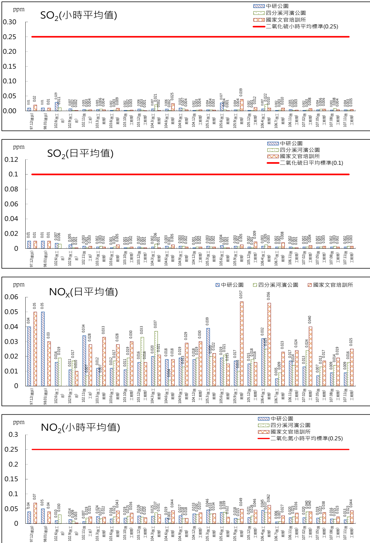
圖 2.1-1 空氣品質監測結果圖(施工期間)(續 1)
