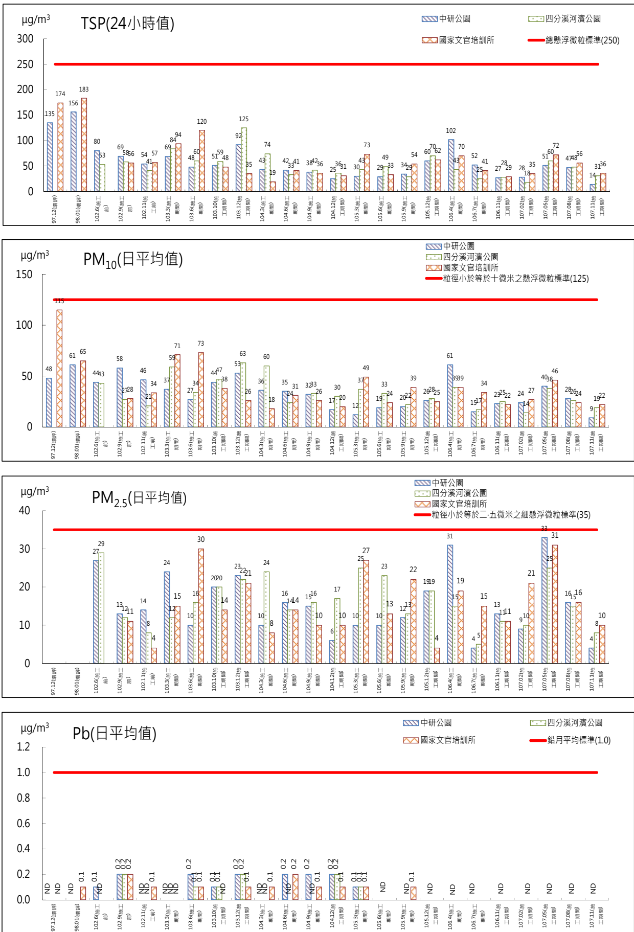
圖 2.1-1 空氣品質監測結果圖(施工期間)
