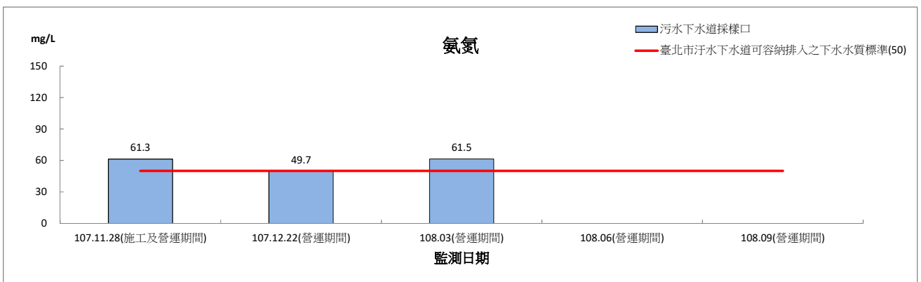
圖 2.7-1 園區污水納管水質監測結果圖(營運期間)(續 6)
