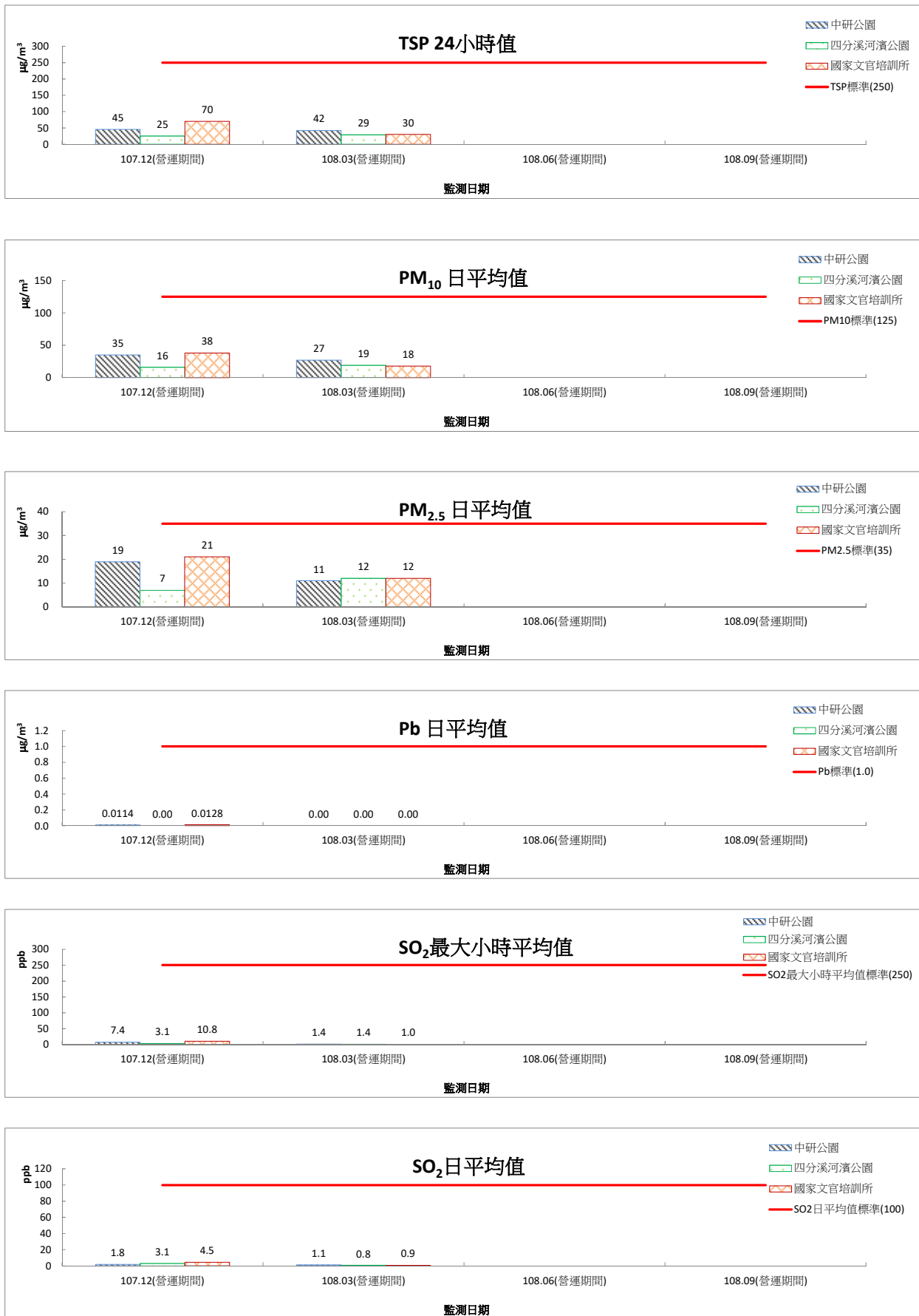
圖 2.1-2 空氣品質監測結果圖(營運期間)
