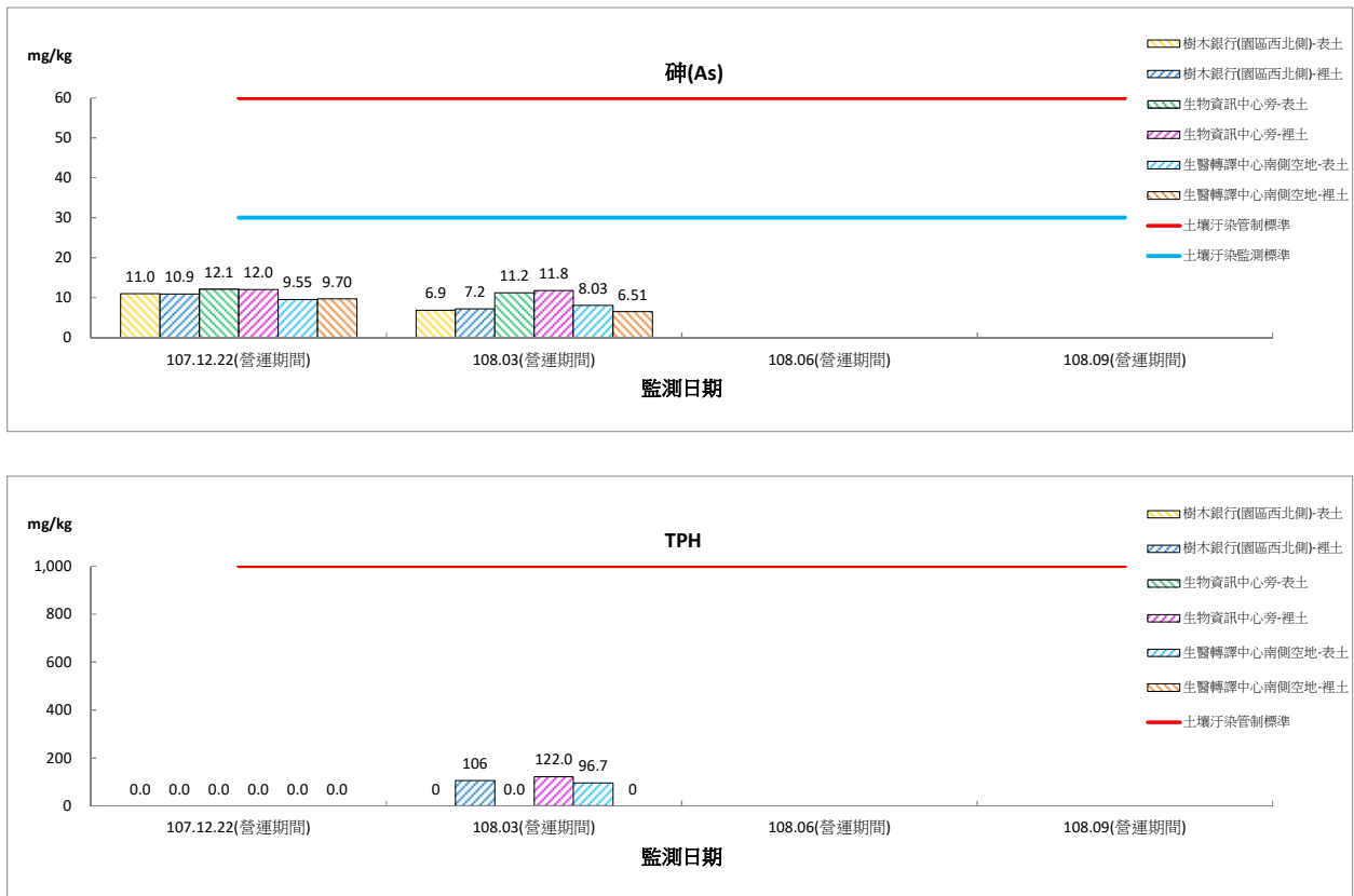
圖 2.3-2 土壤監測結果圖(營運期間)(續 2)
