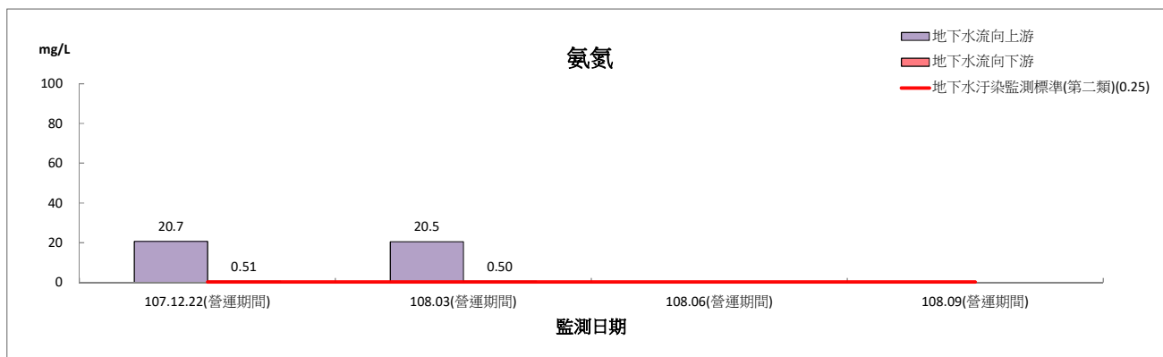
圖 2.5-3 地下水監測結果圖(營運期間)(續 1)
