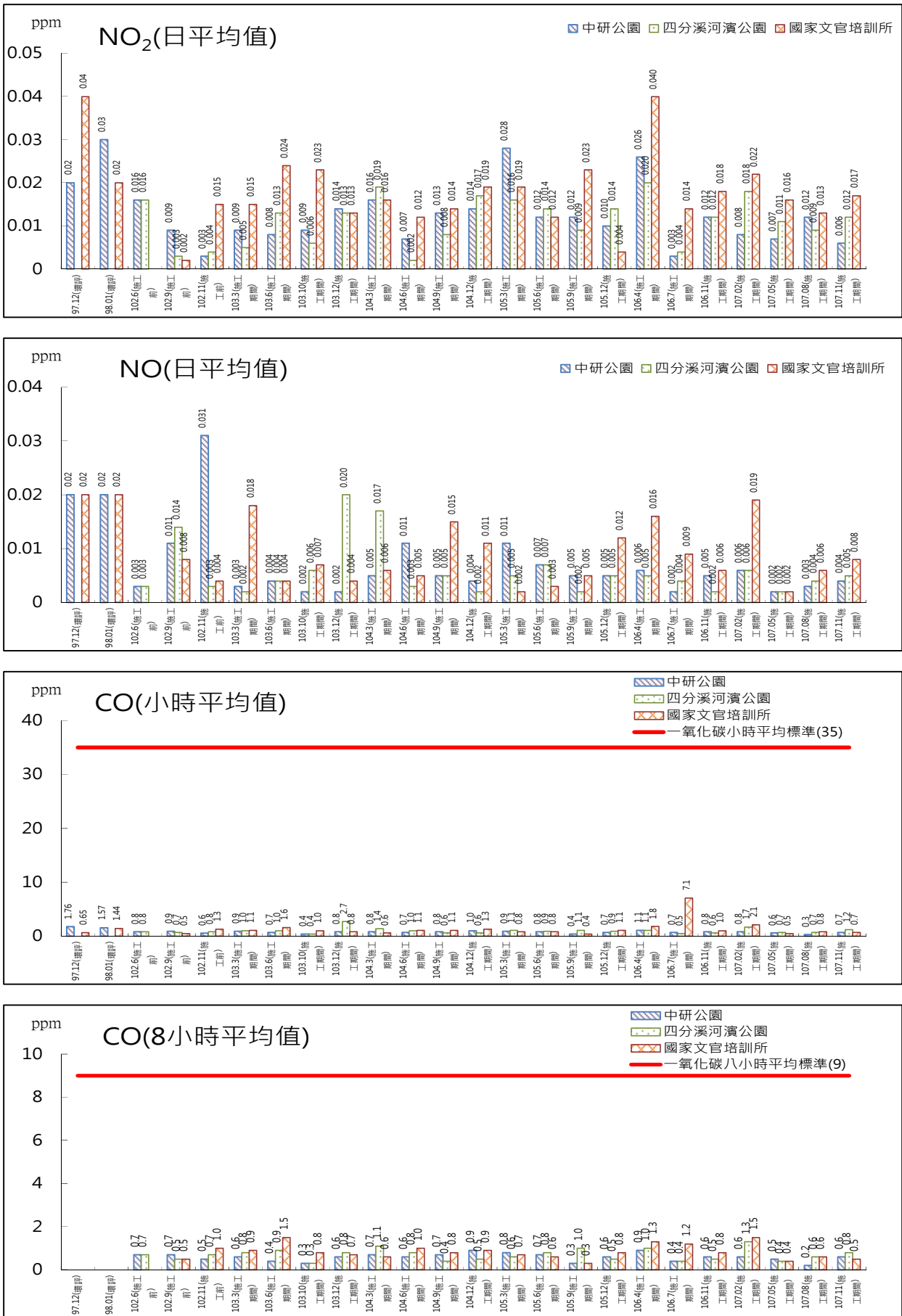
圖 2.1-1 空氣品質監測結果圖(施工期間)(續 2)
