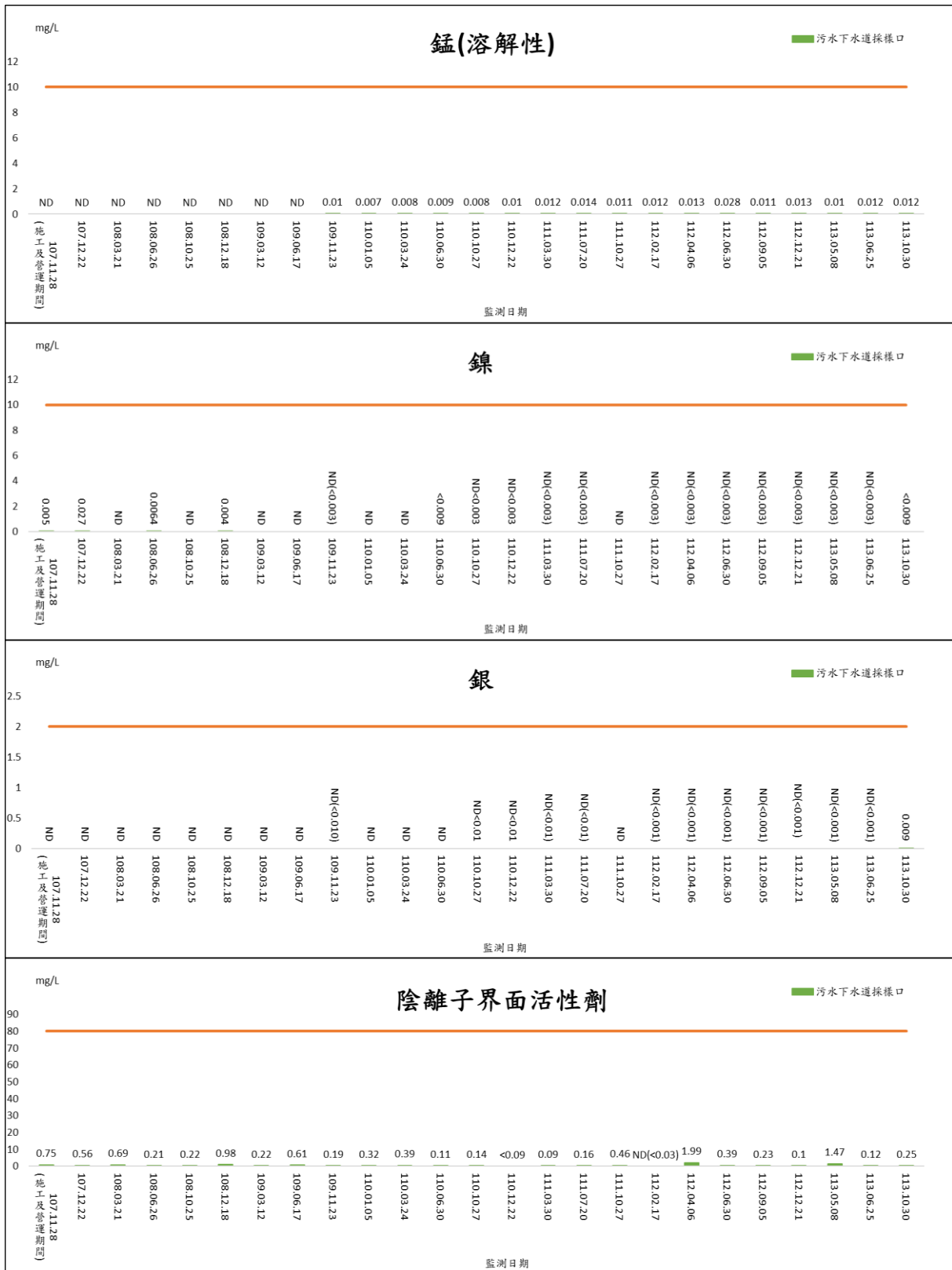
圖 2.7-1 園區污水納管水質監測結果圖(營運期間)(續 5)
