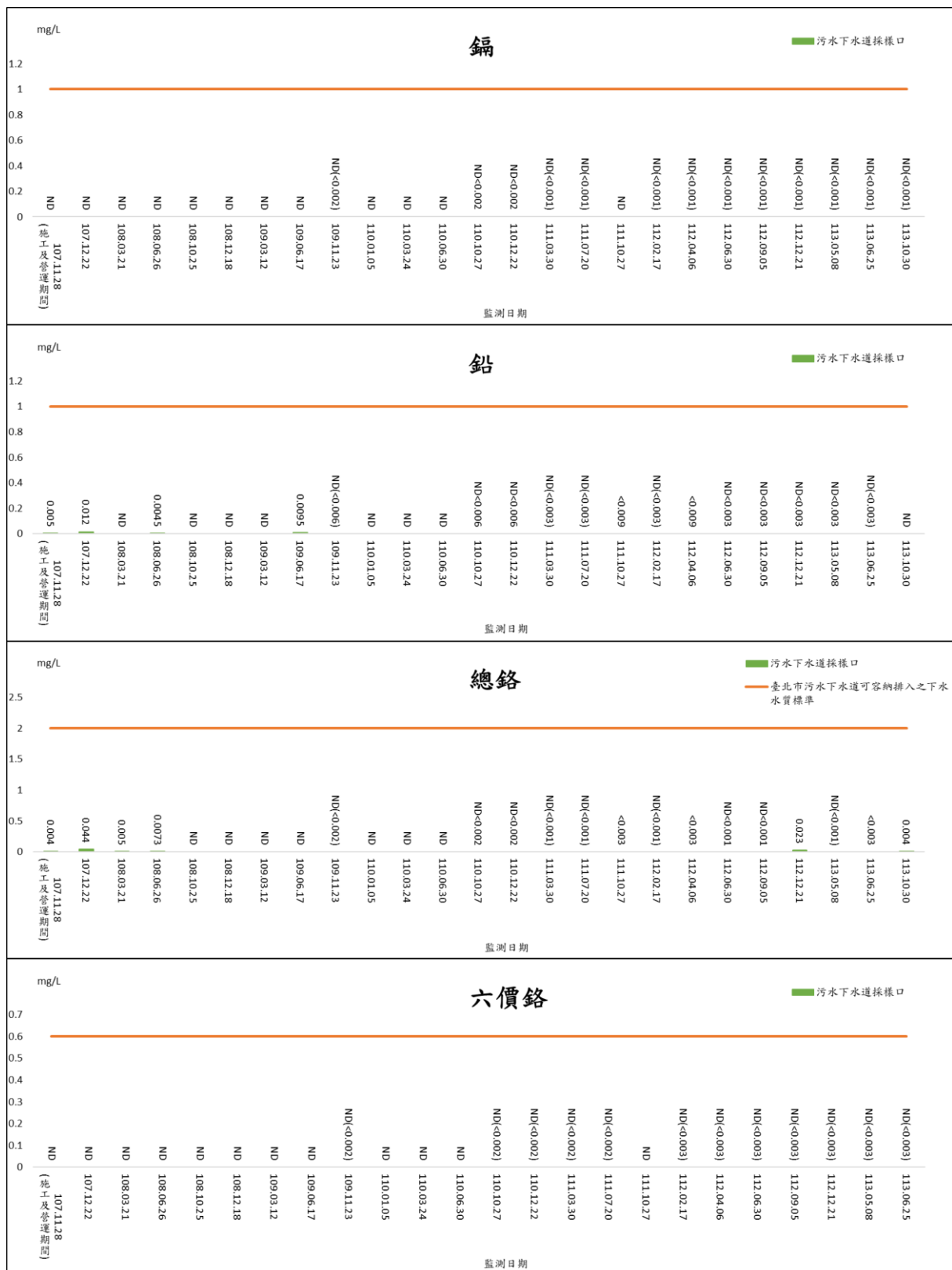
圖 2.7-1 園區污水納管水質監測結果圖(營運期間)(續 3)
