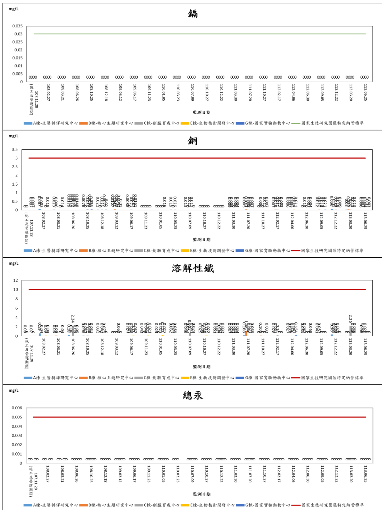
圖 2.8-1 實驗室廢水納管水質監測結果圖(營運期間)(續 3)
