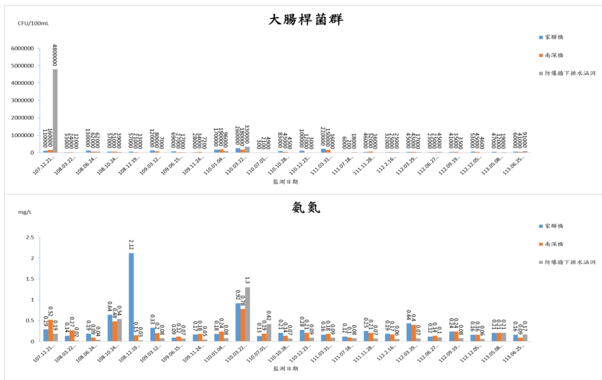
圖 2.4-3 地面水質監測結果圖(營運期間)(續 2)
