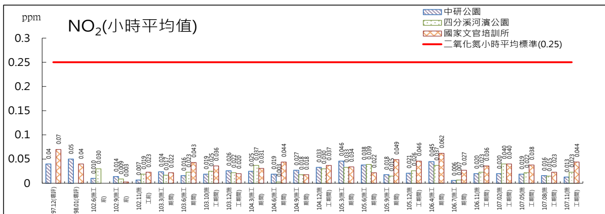
圖 2.1-2 空氣品質監測結果圖(施工期間)(續 1)
