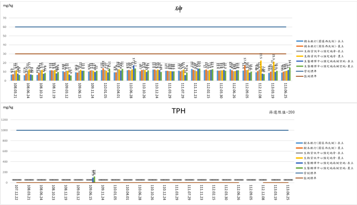
圖 2.3-2 土壤監測結果圖(營運期間)(續 2)
