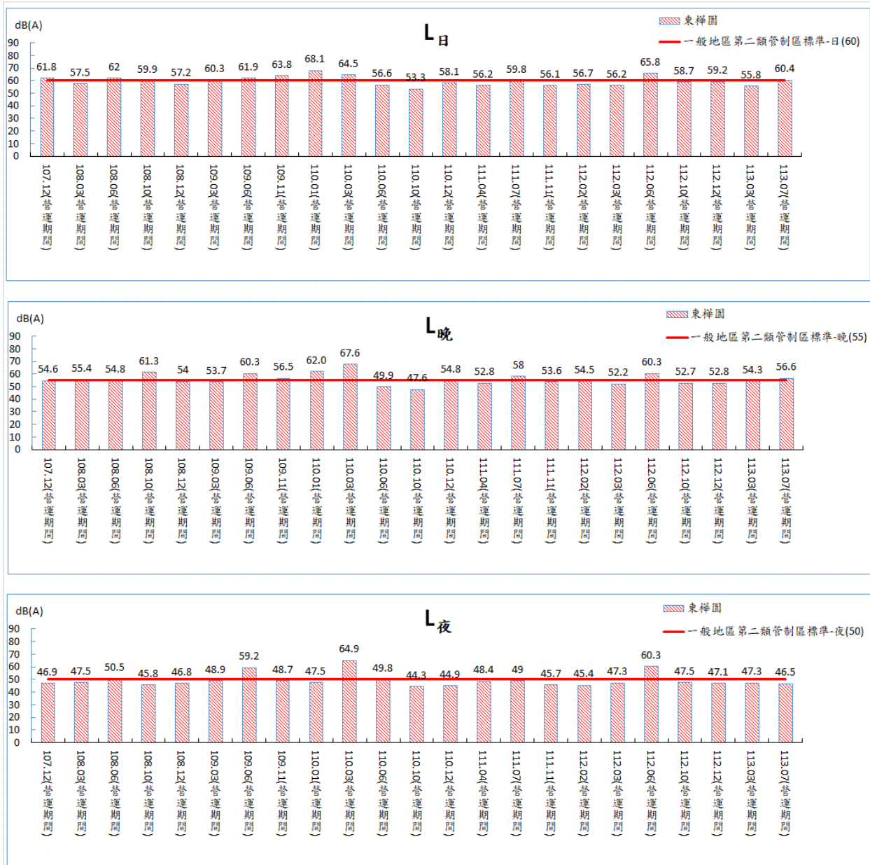
圖 2.2.1-2 東樺園噪音監測結果圖(營運期間)
