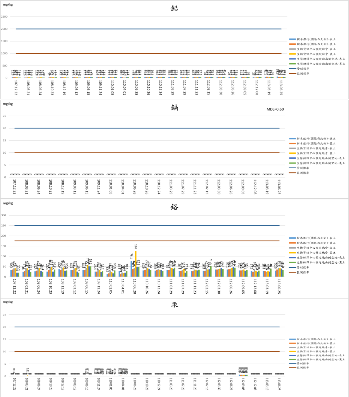
圖 2.3-2 土壤監測結果圖(營運期間)(續 1)
