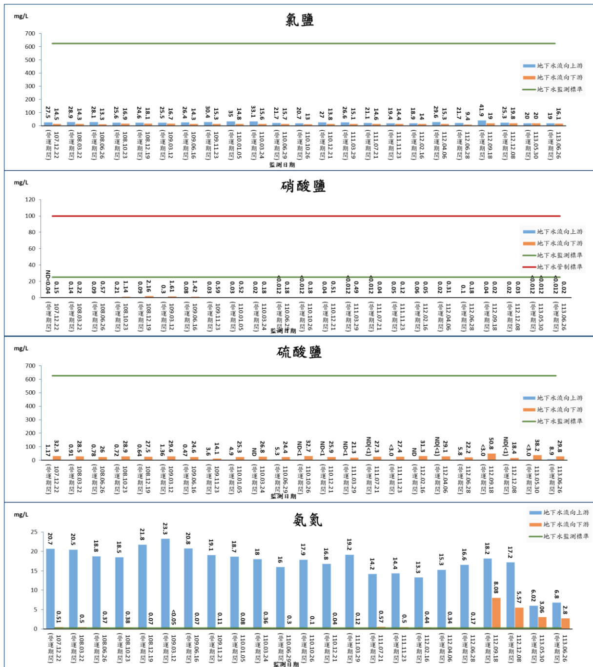
圖 2.5-3 地下水監測結果圖(營運期間)(續 1)
