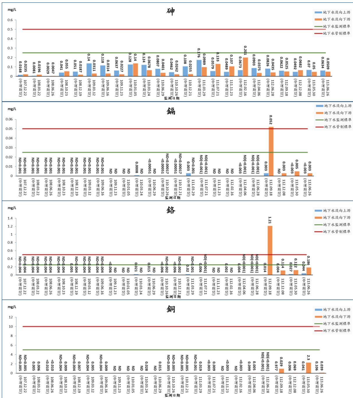
圖 2.5-3 地下水監測結果圖(營運期間)(續 3)
