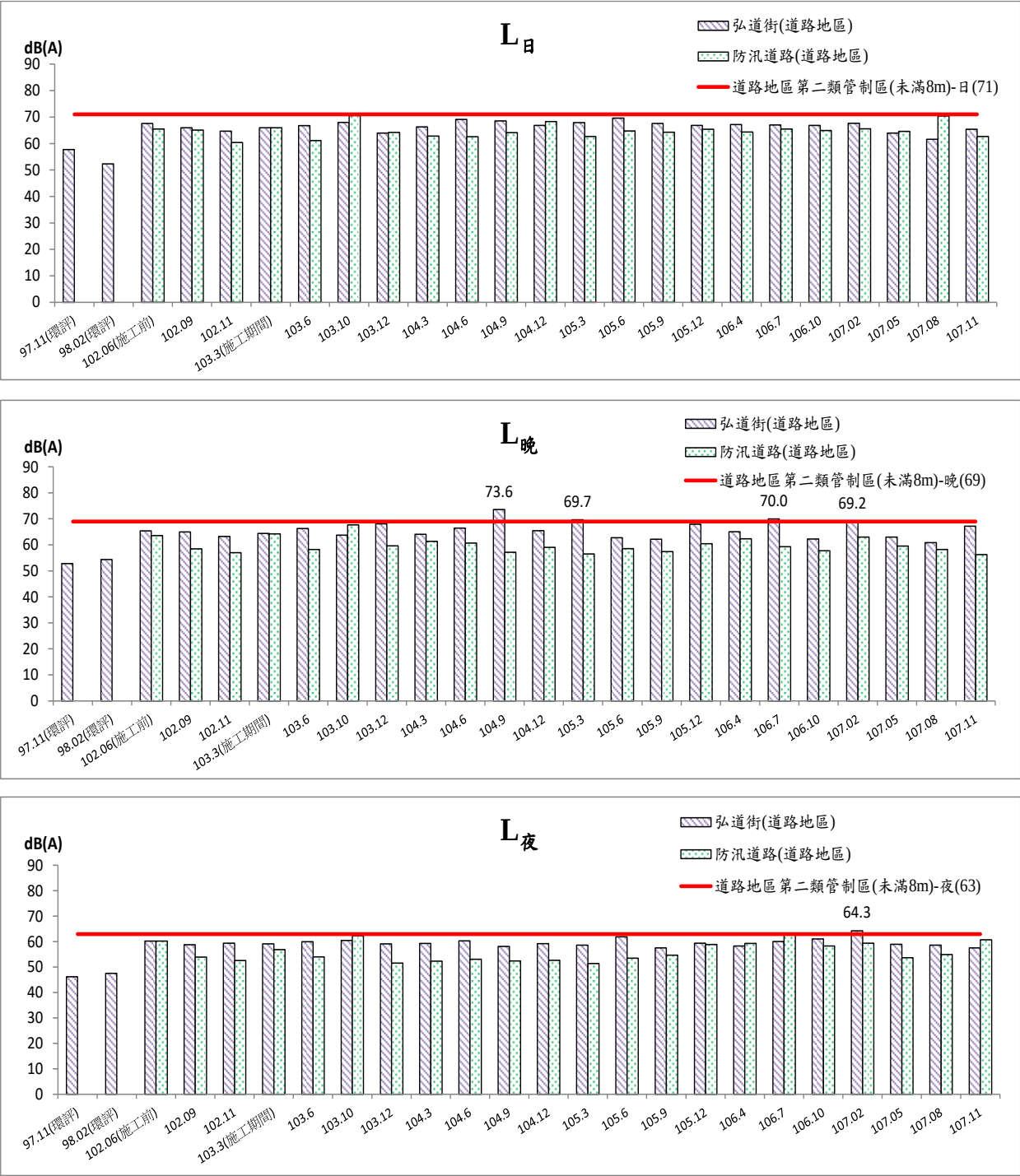
圖 2.2.1-3 防汛道路噪音監測結果圖(施工期間)
