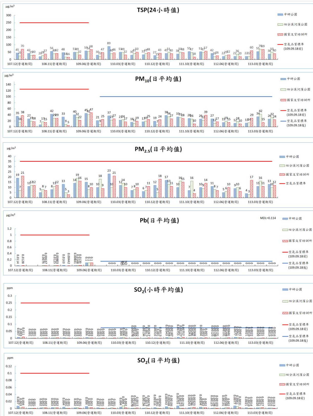
圖 2.1-3 空氣品質監測結果圖(營運期間)
