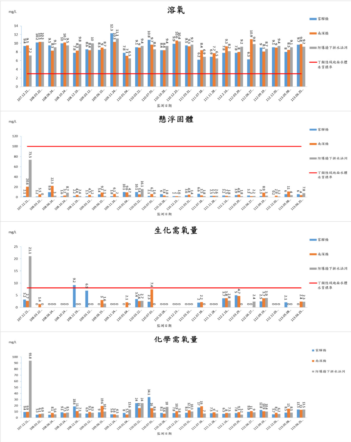
圖 2.4-3 地面水質監測結果圖(營運期間)(續 1)
