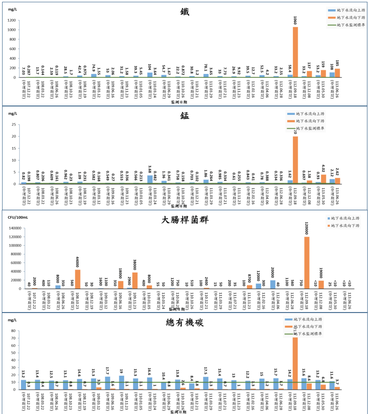
圖 2.5-3 地下水監測結果圖(營運期間)(續 2)
